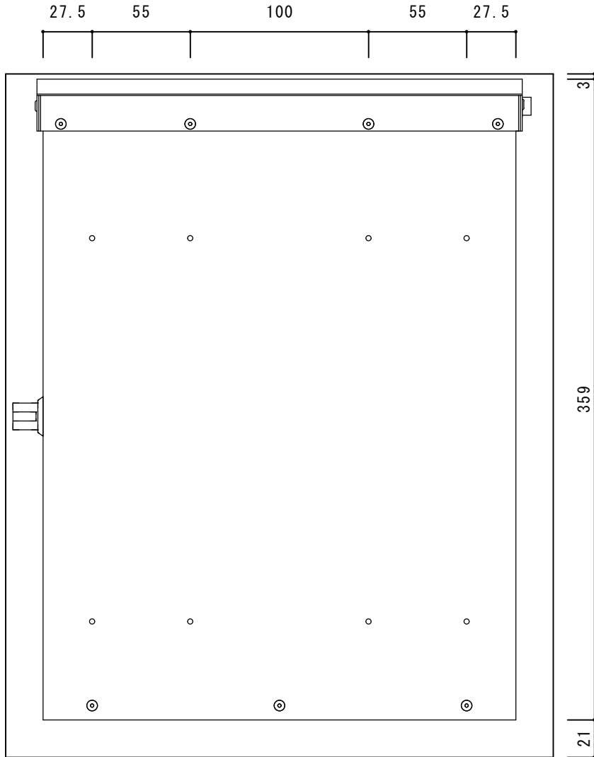
【背面図】
