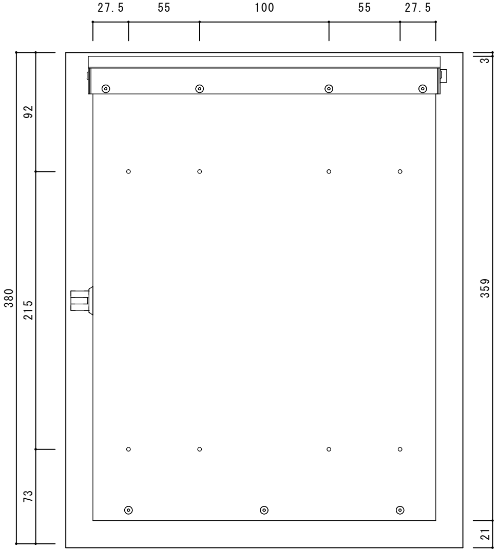
【背面図】
