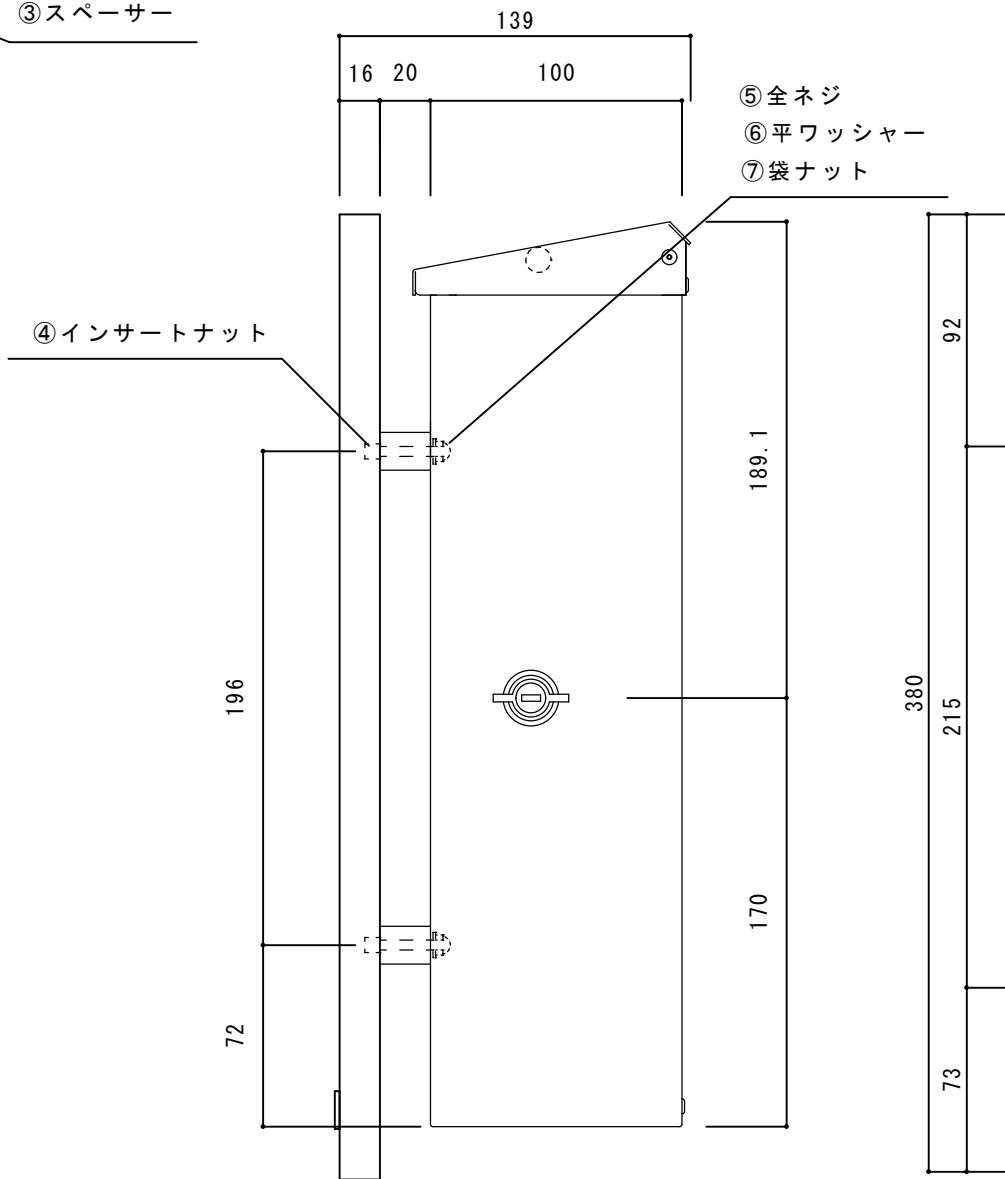
【側面図】
