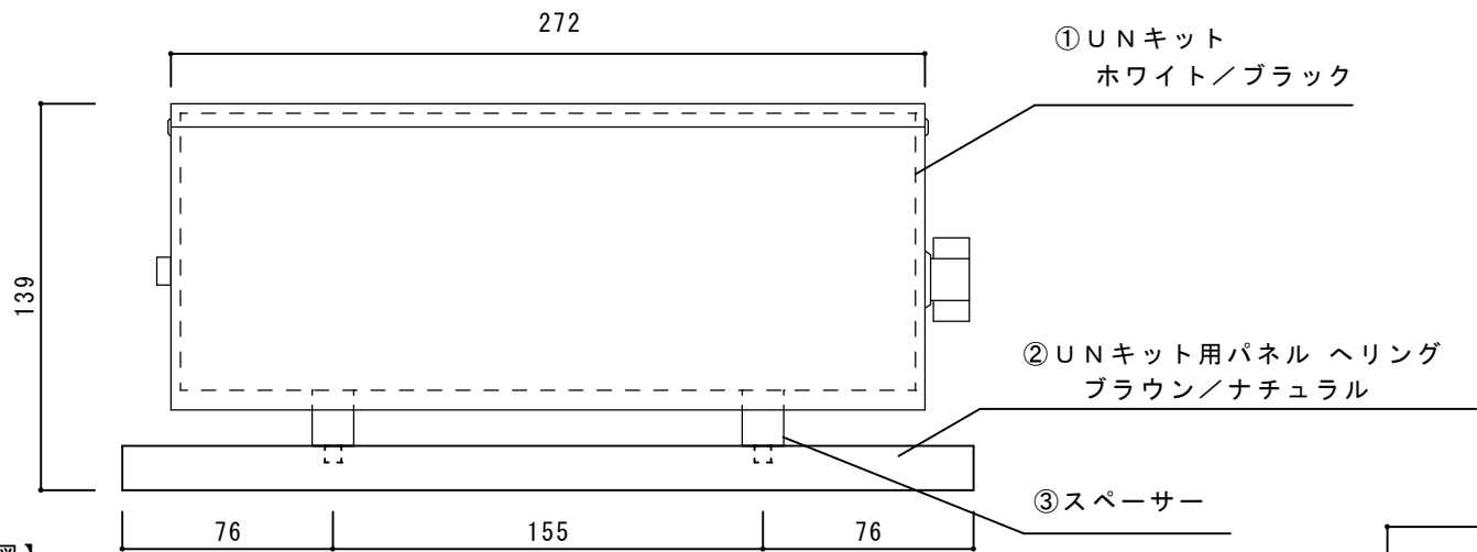
【上面図】
