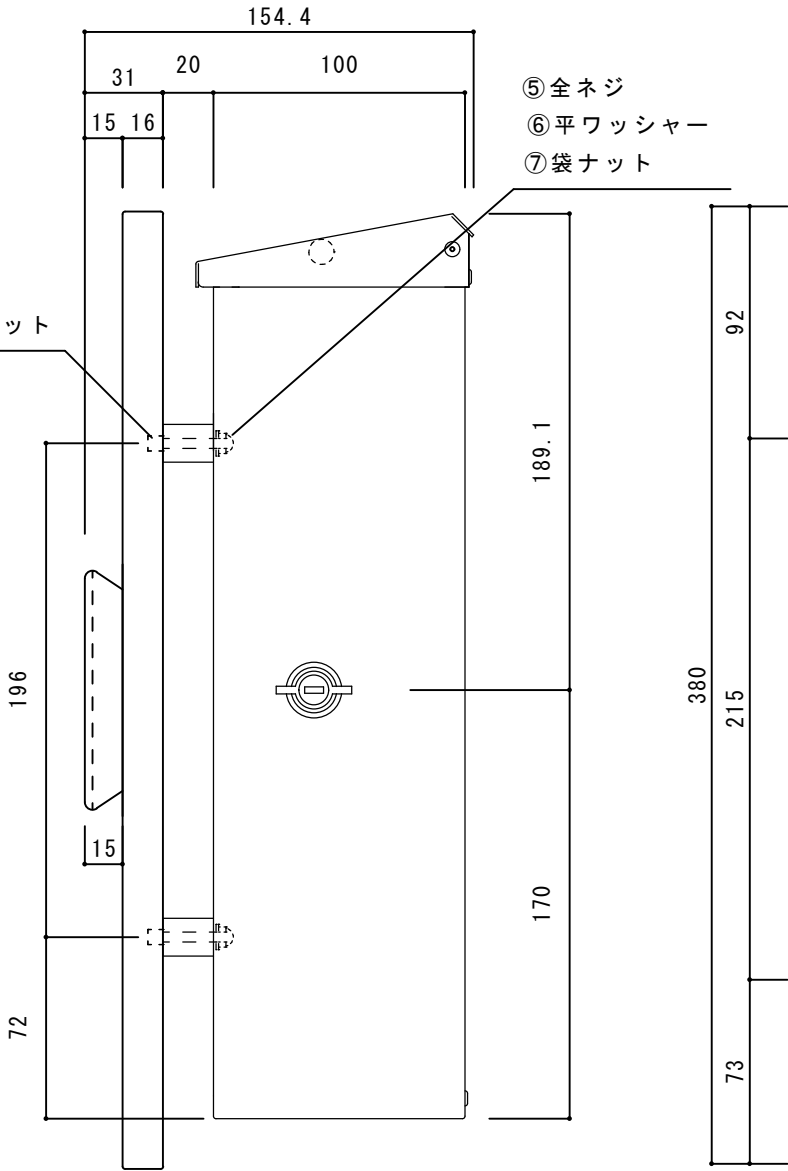
【側面図】
