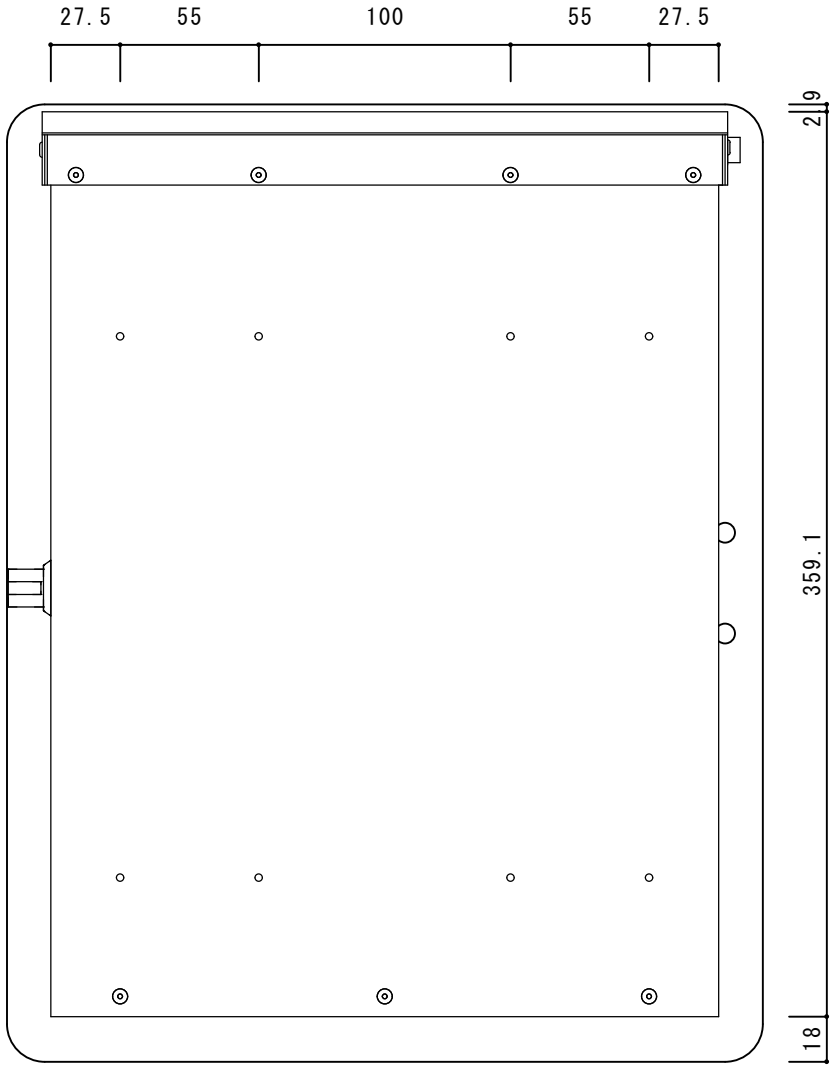
【背面図】
