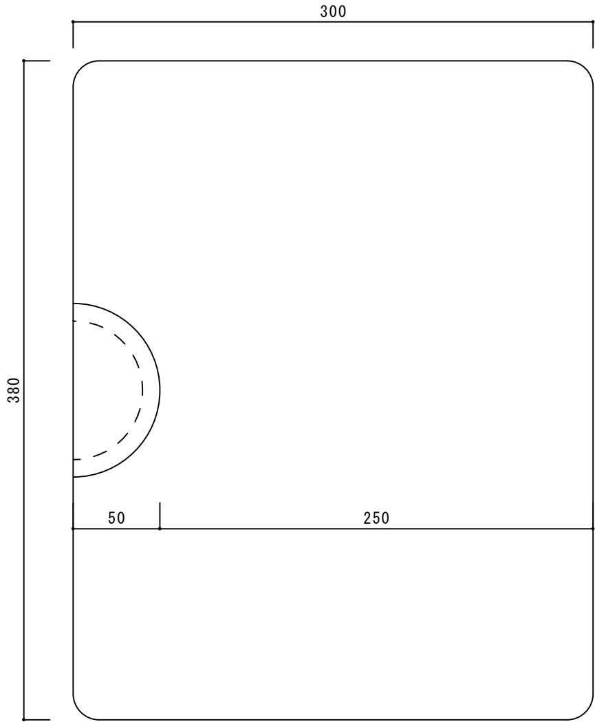
【正面図】
