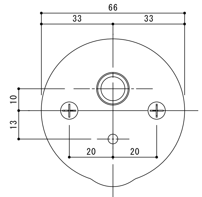
背面図
