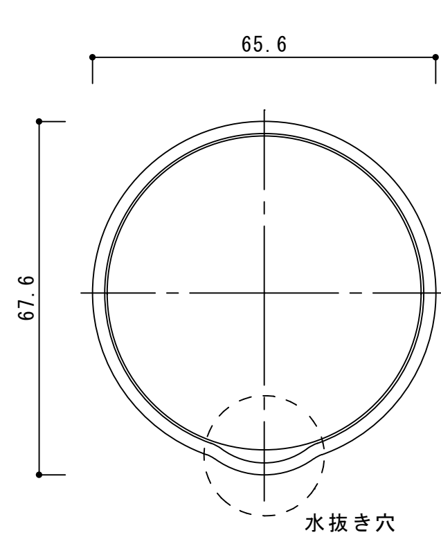
上面図
