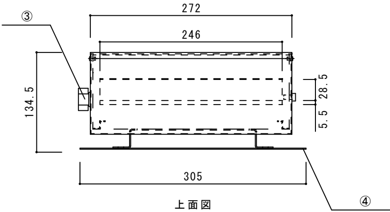
上面図
