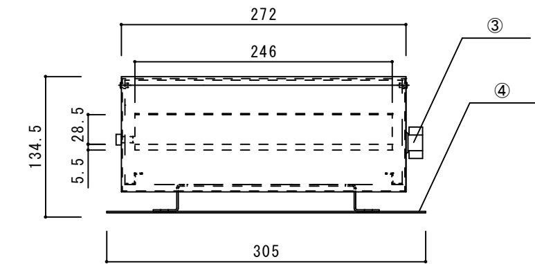
上面図
