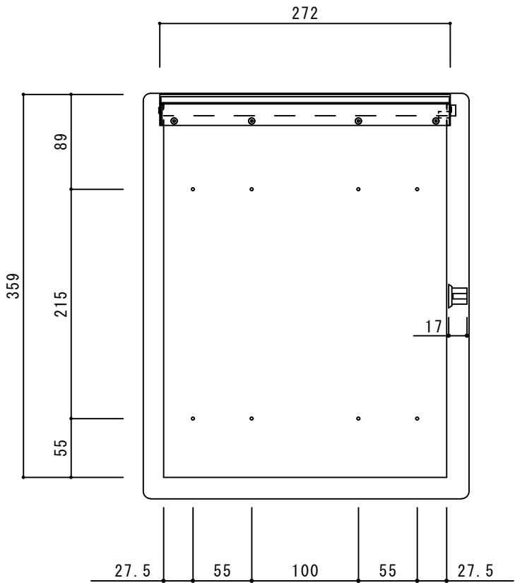
背面図
