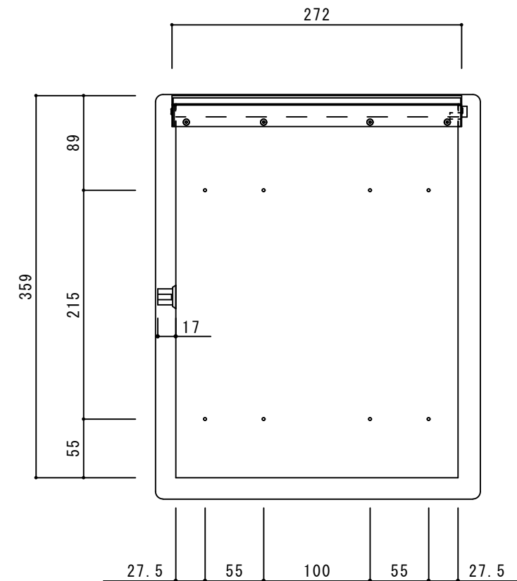
背面図
