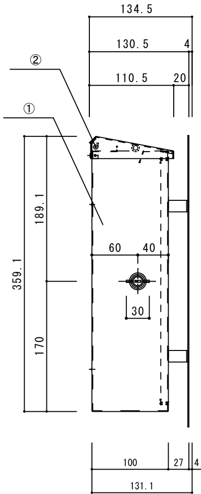
側面図
