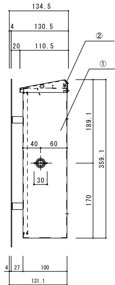
側面図
