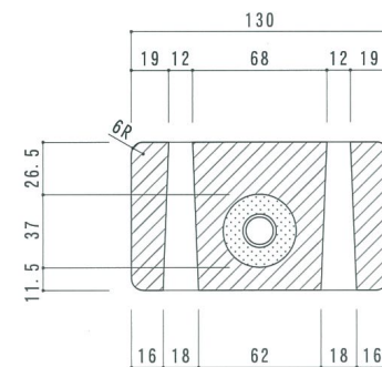
B - B' 断面図 (S = 1 / 3)
