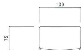
上面図
