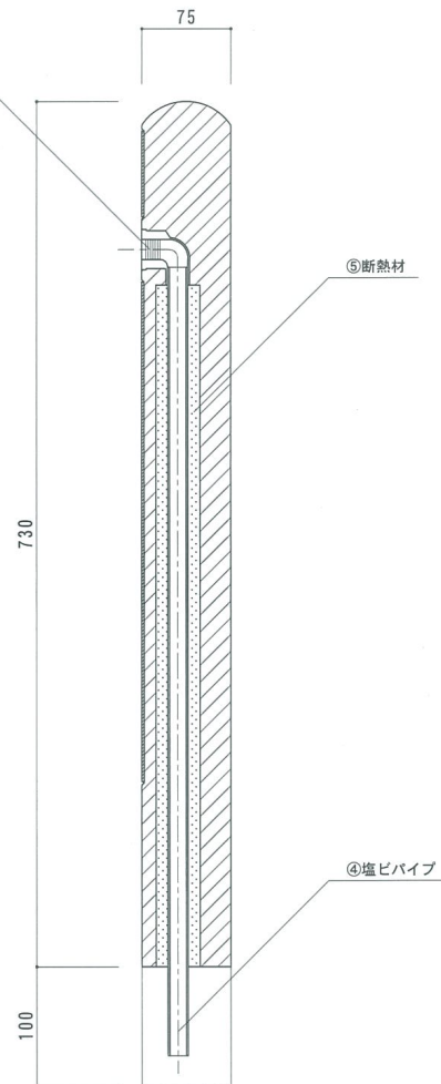
右側面 断面図
