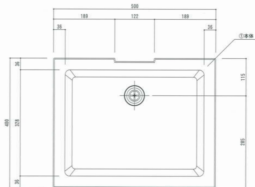
上面図
