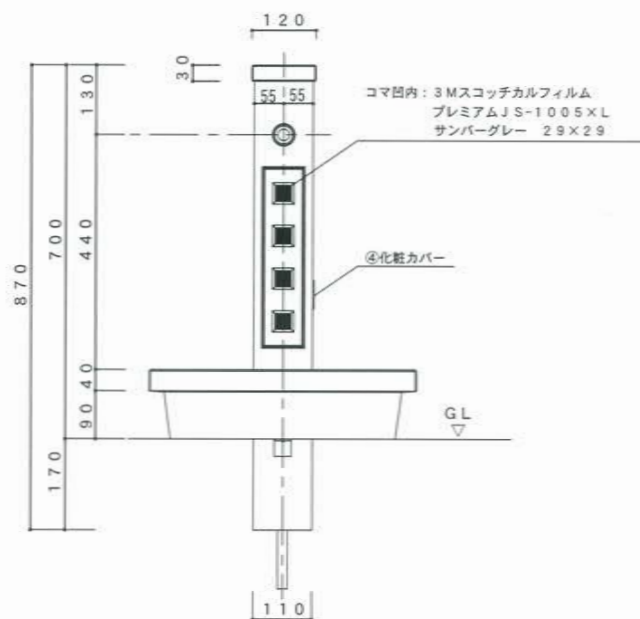
正面図
