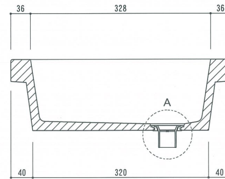
側断面図
