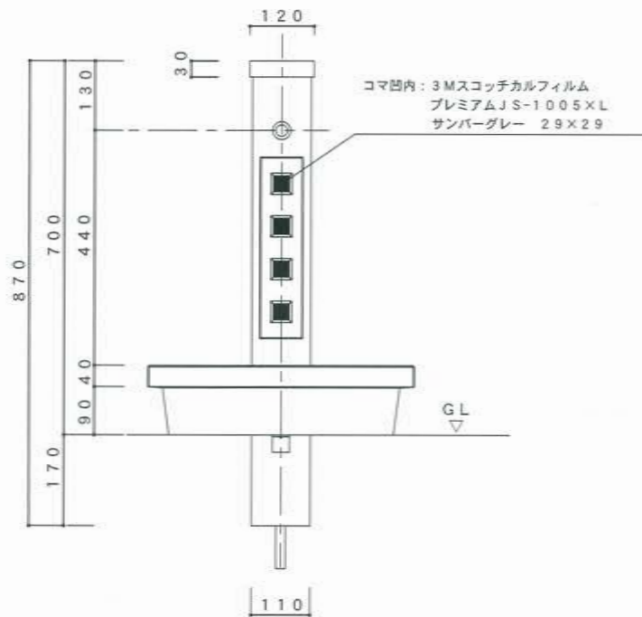
正面図
