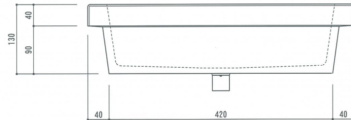
正面図
