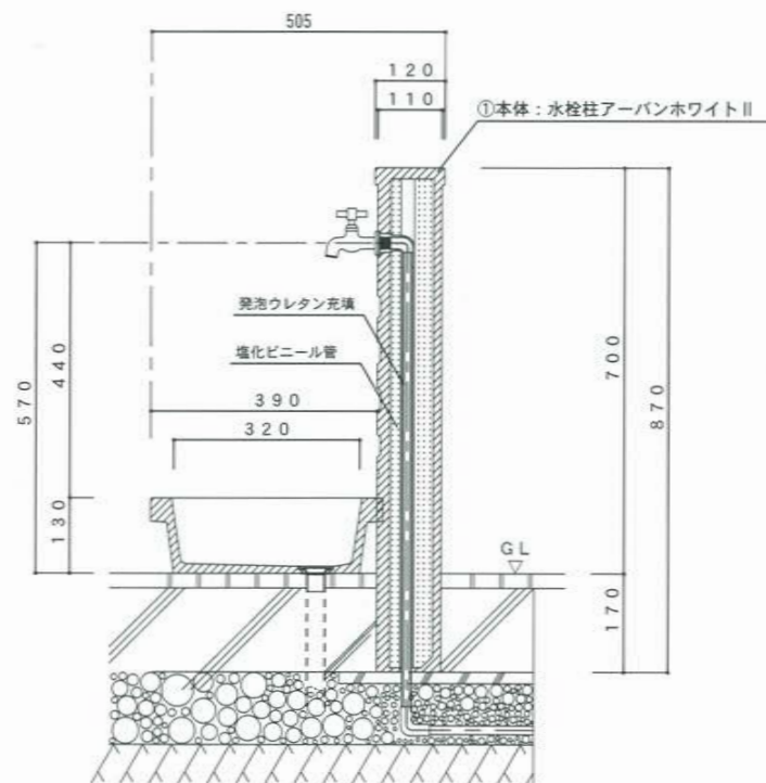
断面図
