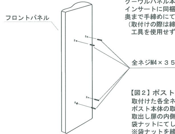
【図1】全ネジの取付け
