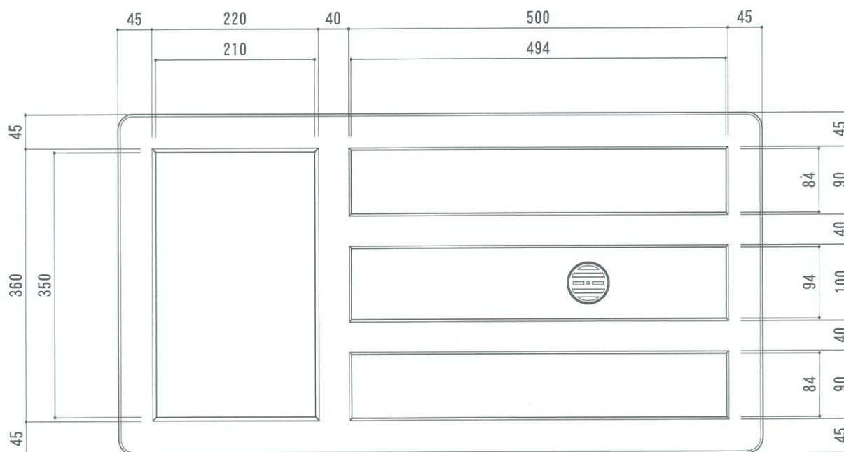
底面図
