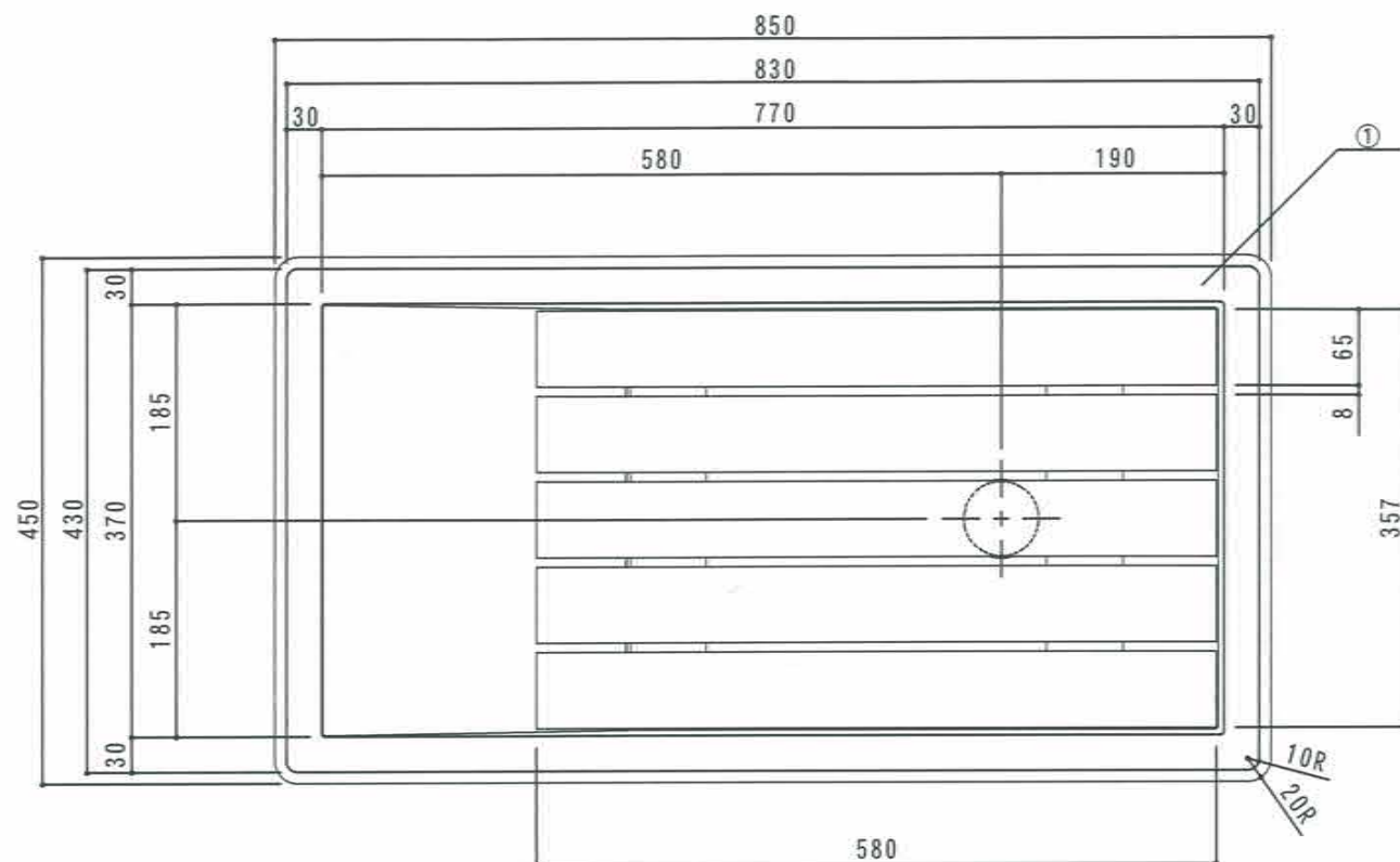
上面図
