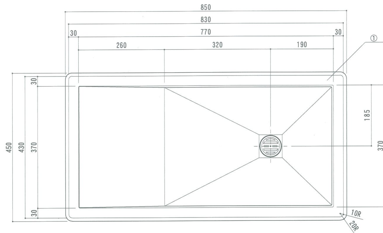
上面図
