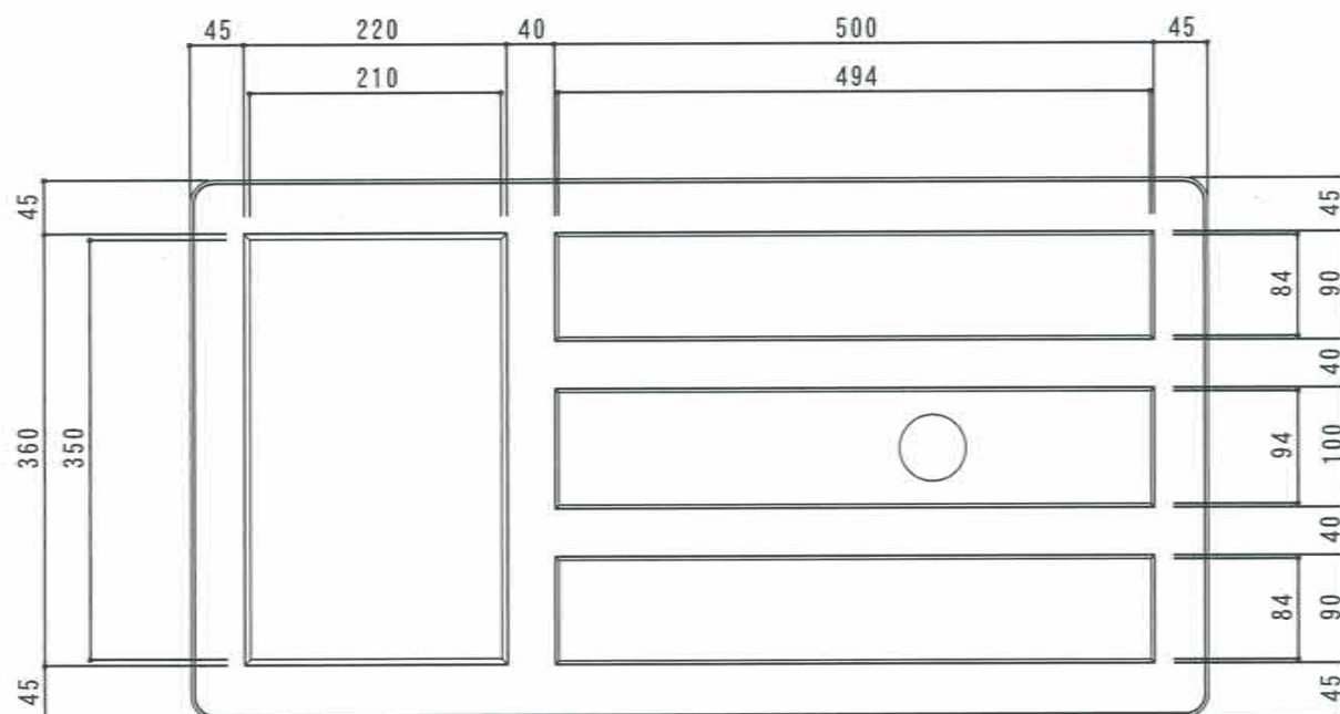
底面図
