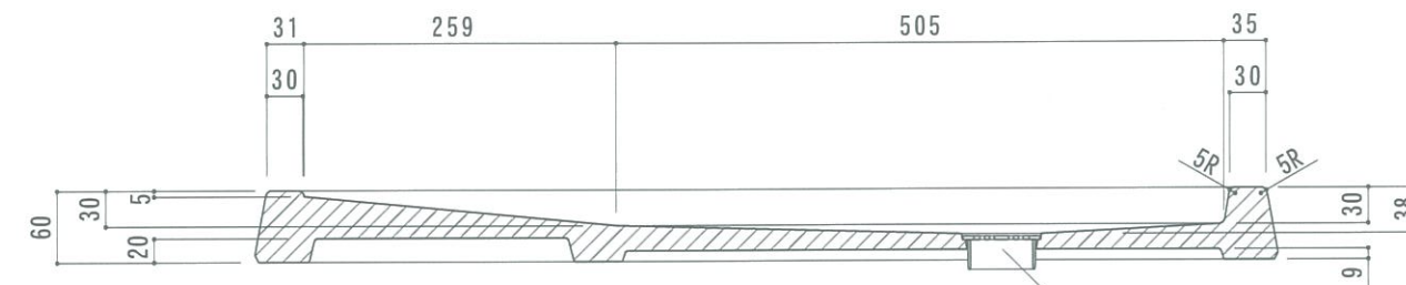
正面断面図
