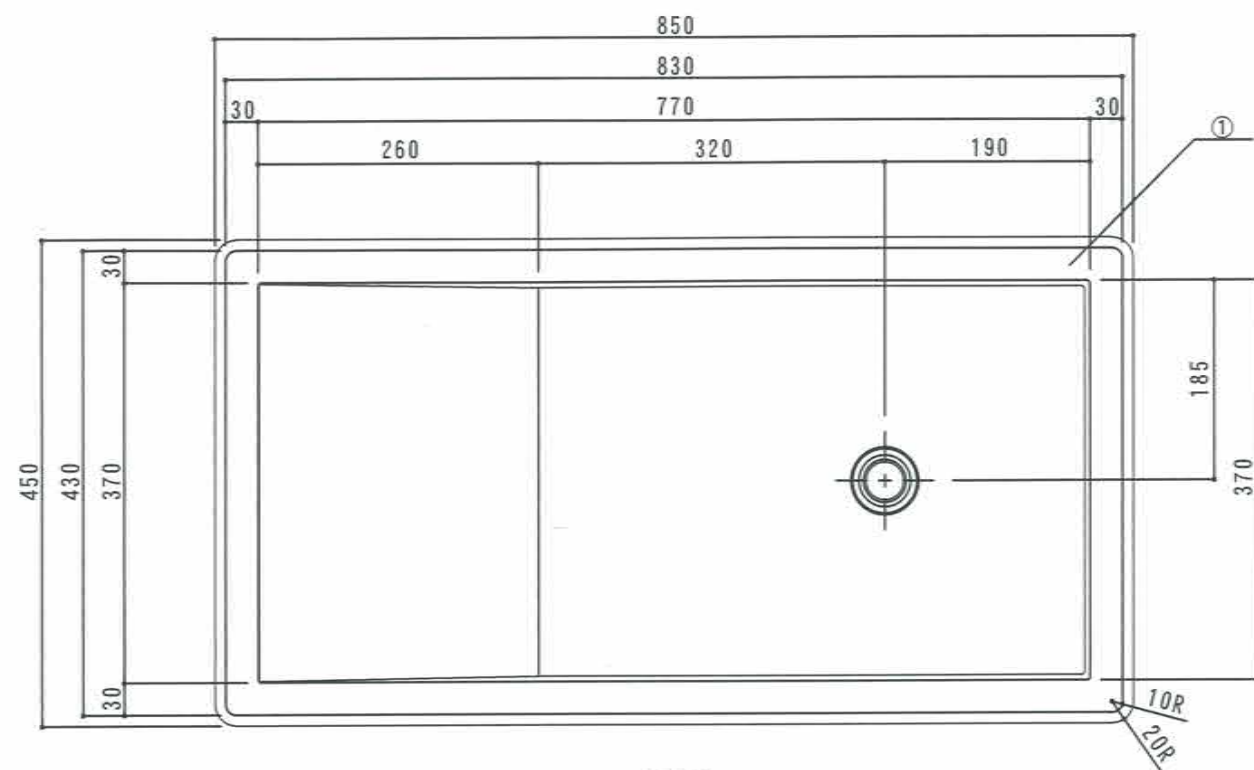
上面図
