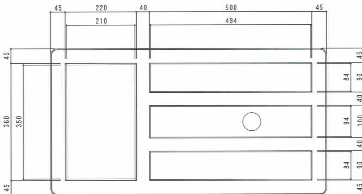
底面図
