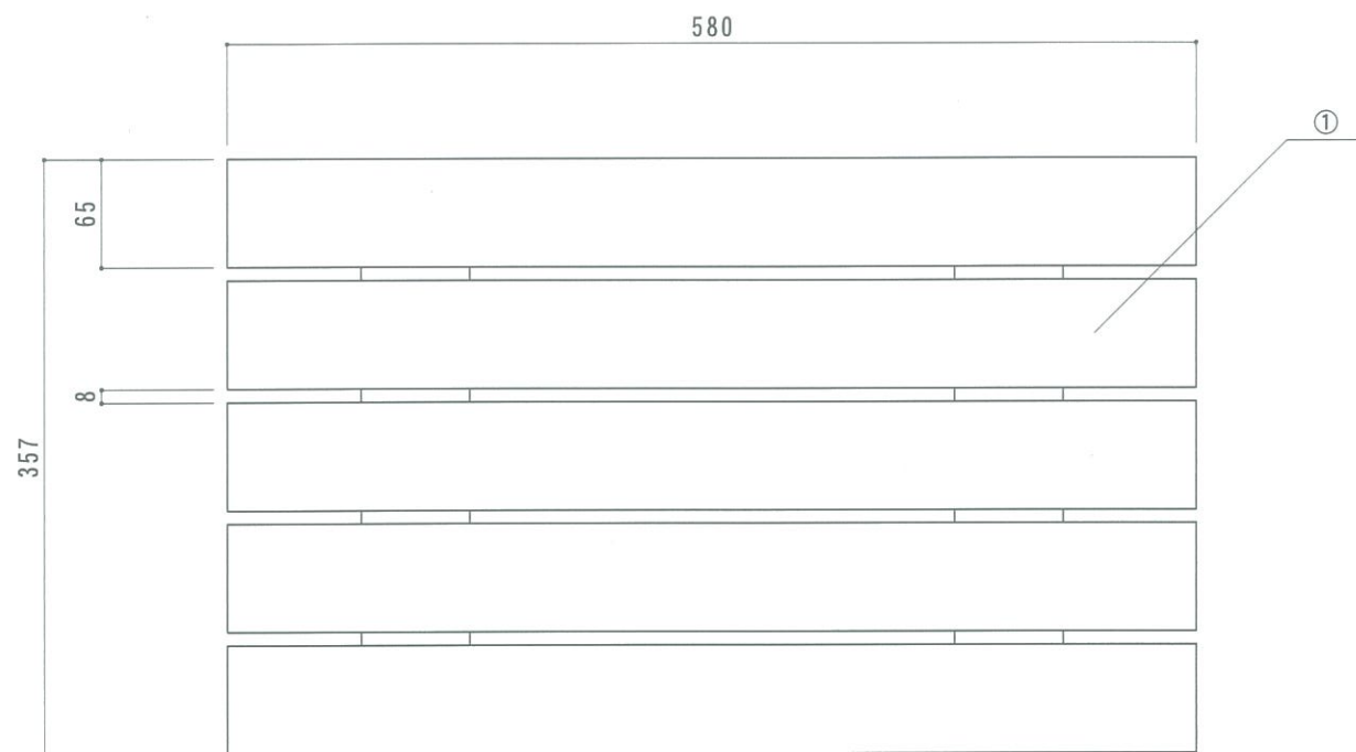
上面図
