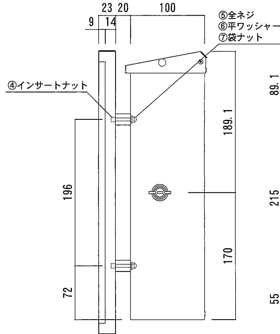
【側面図】
