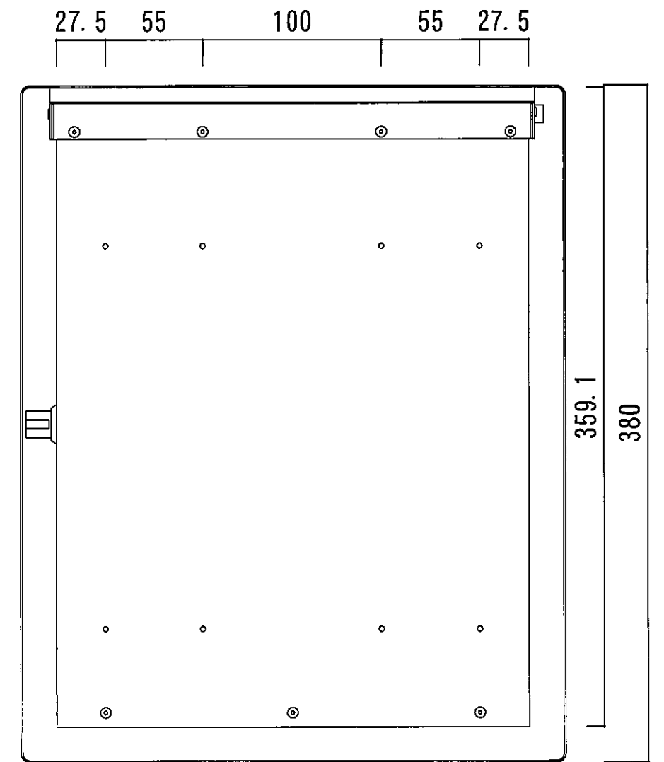
【背面図】
