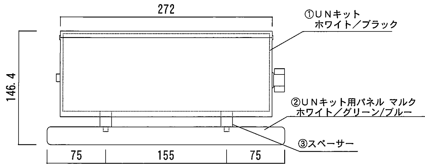
【上面図】
