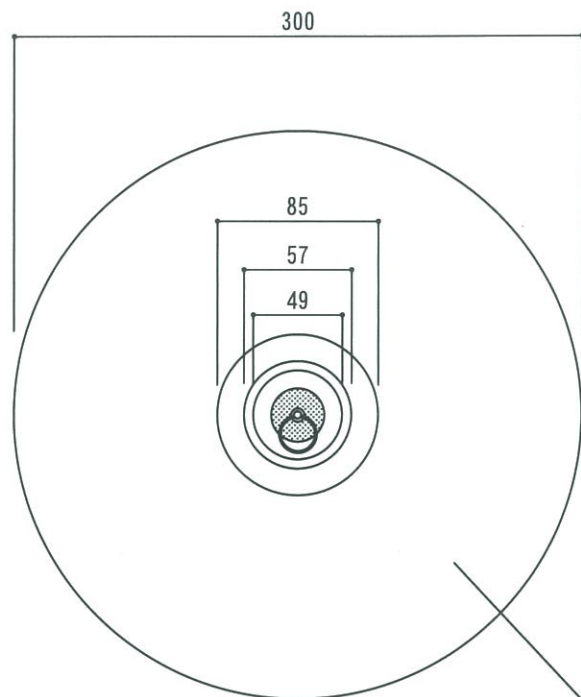
上面図
