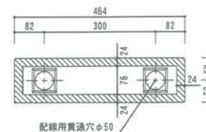
A'-A 断面図
