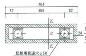
A'-A断面図
