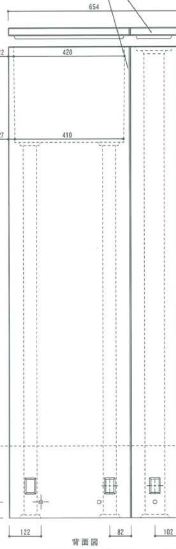
背面図
