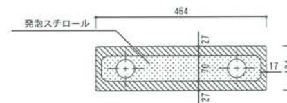
B'-B 断面図
