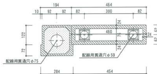
A'-A断面図
