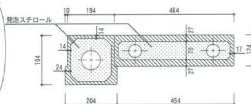
B'-B断面図
