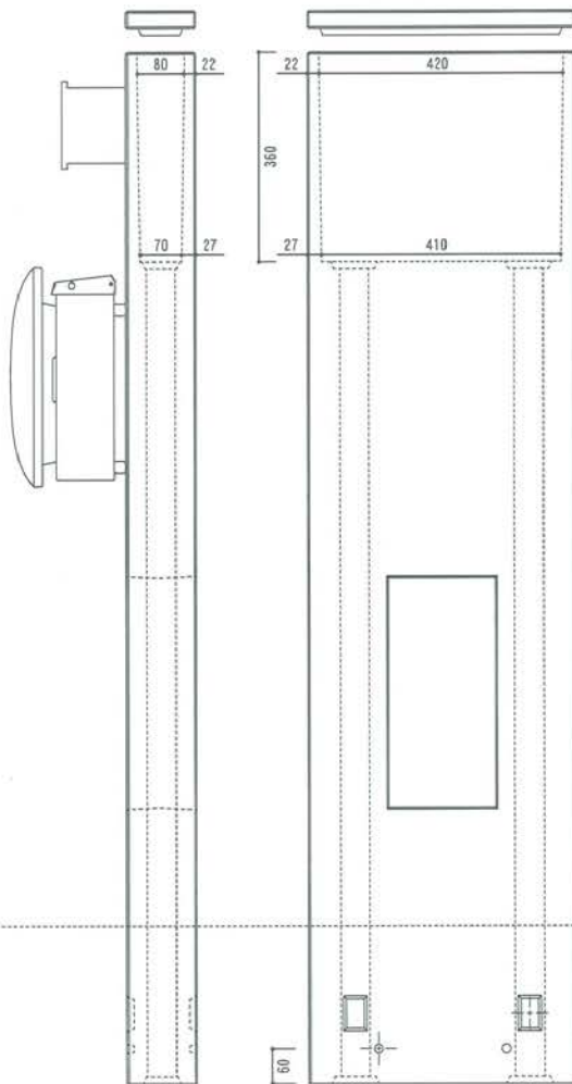
背面図
