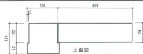
上面図
