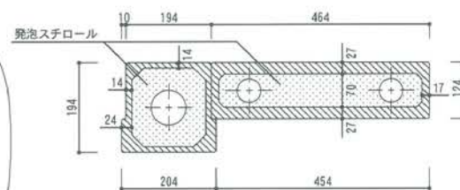
B'-B断面図
