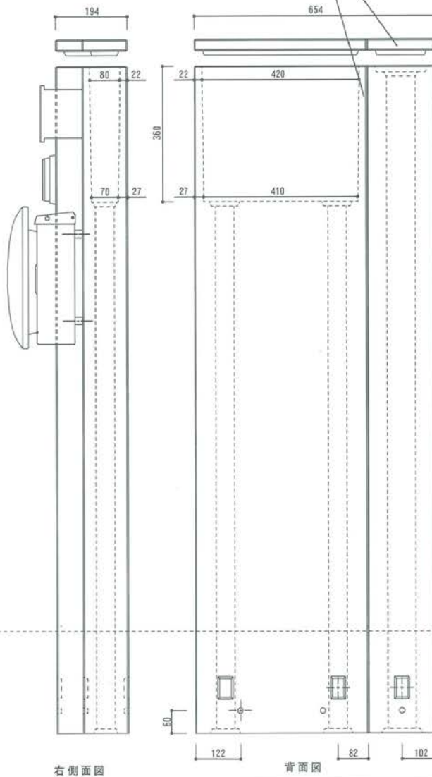
右側面図
