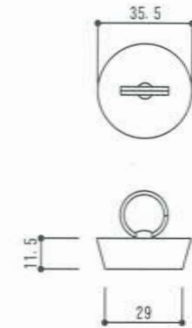
△ ③ゴム栓 (S=1/2)
