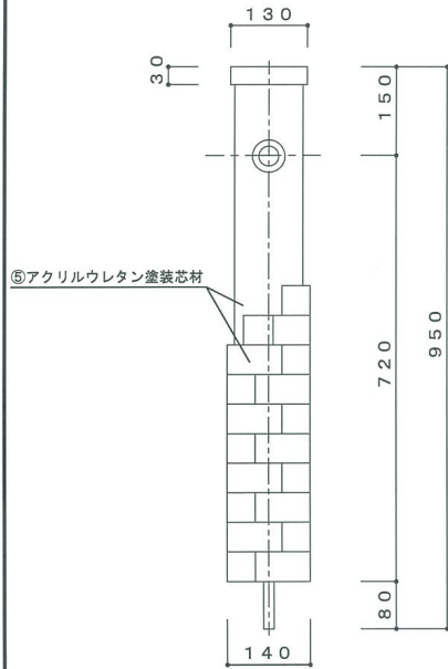
正面図
