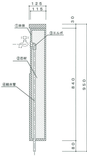
側断面図
