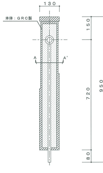
前断面図
