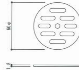
②排水目皿 (S=1/2)
