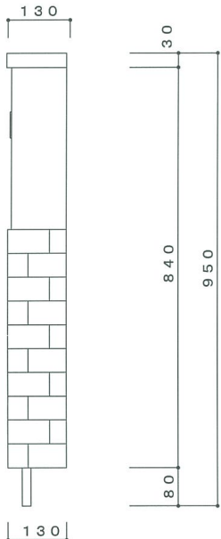
側面図
