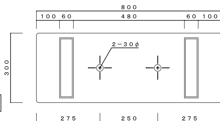
底面図
