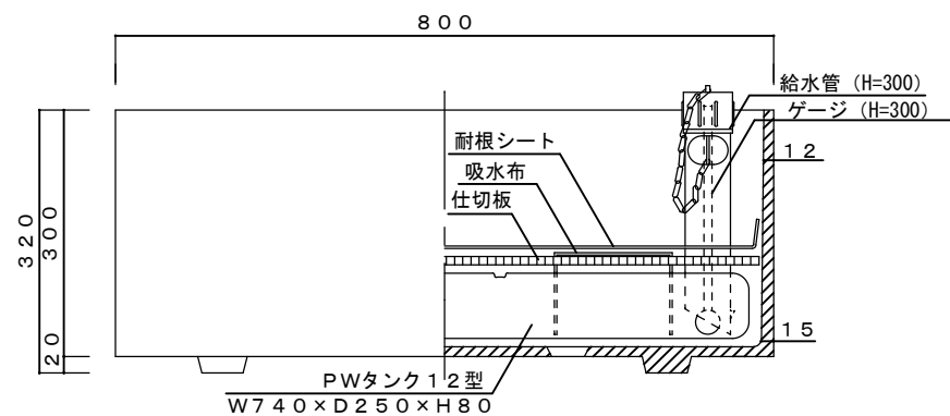
立・断面図
