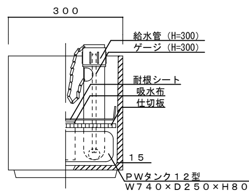
側・断面図
