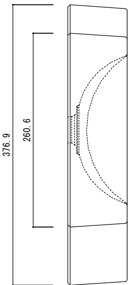
【側面図】
