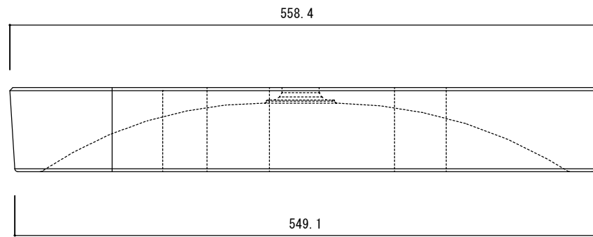
【正背面図】
