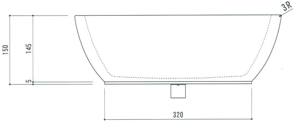
正面図
