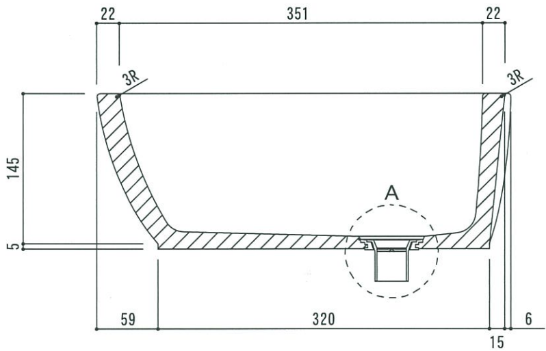
側断面図
