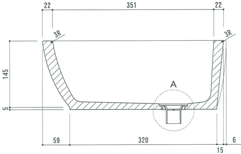
側断面図
