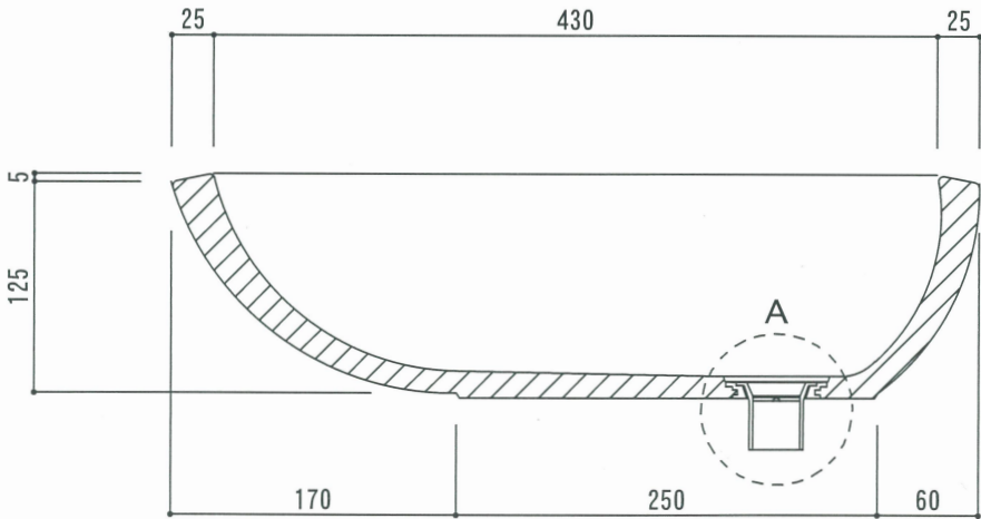
側断面図
