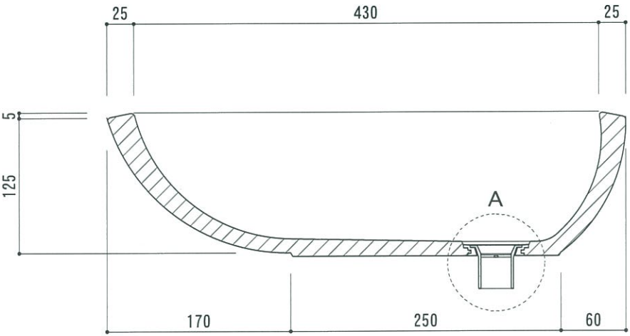
側断面図
