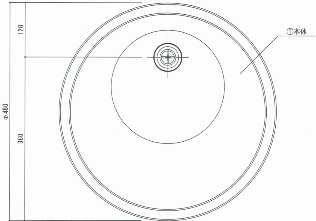
上面図
