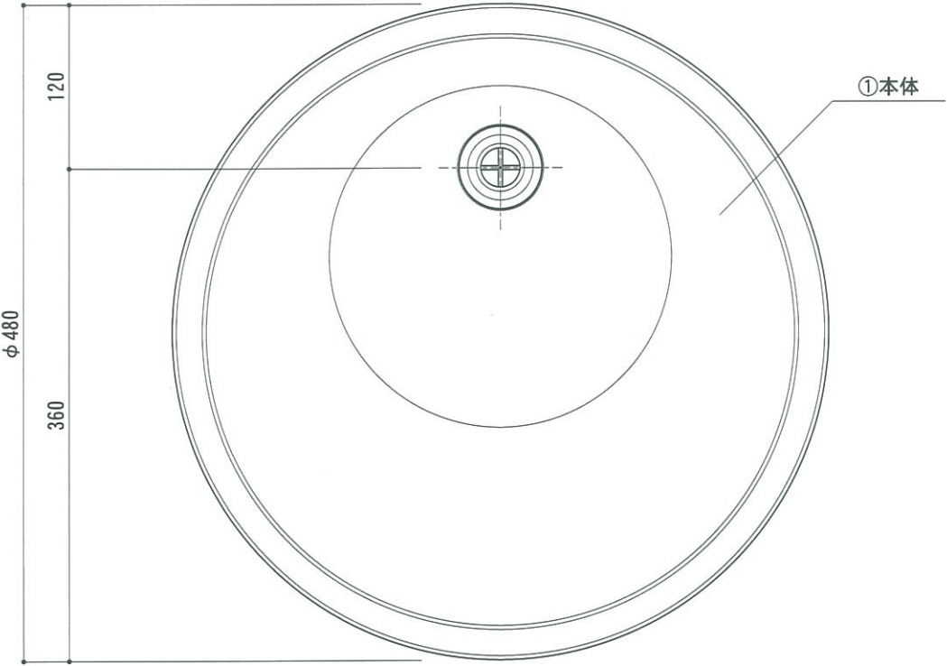
上面図
