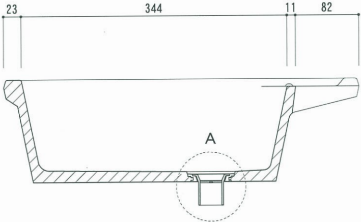
側断面図
