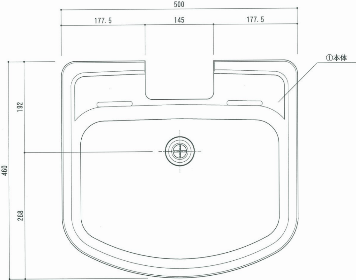
上面図
