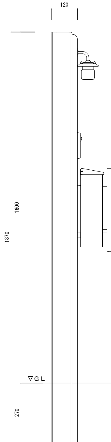
【左側面図】
