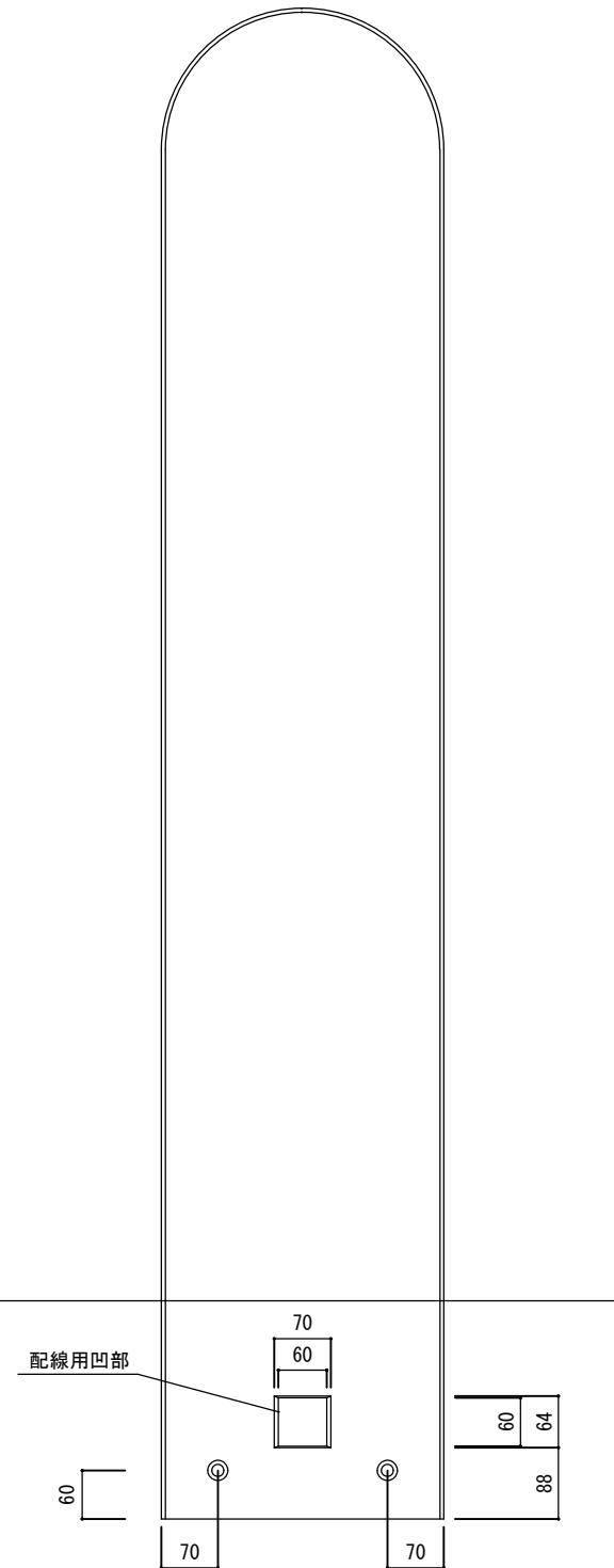
【背面図】
