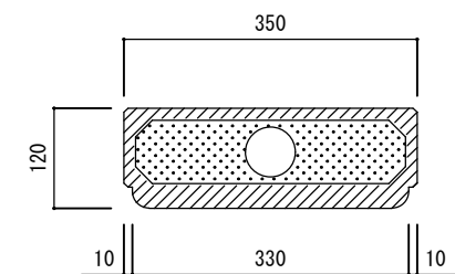
【B-B' 断面図】
