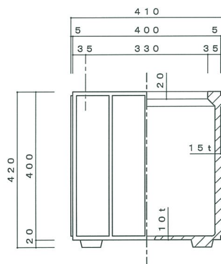
立・断面図
