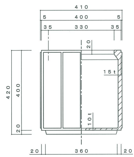
側・断面図
