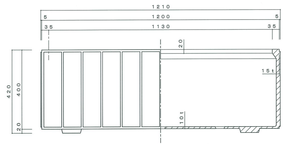
立・断面図
