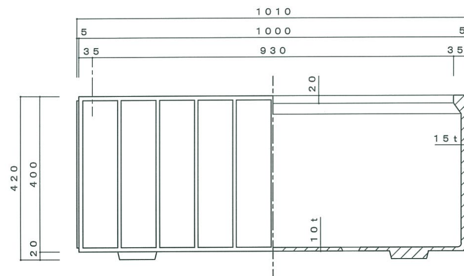
立・断面図
