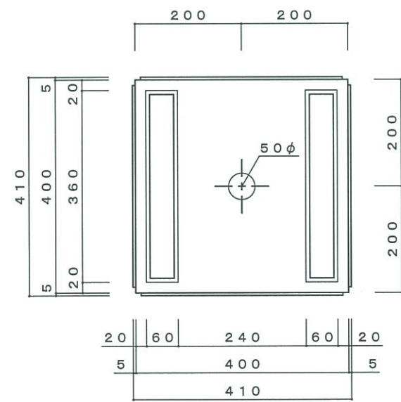
底面図
