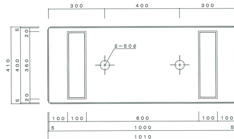
底面図
