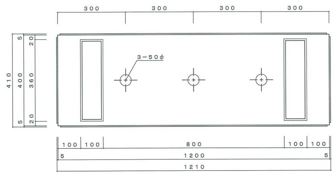
底面図
