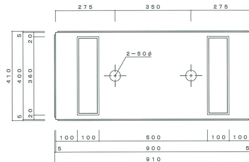
底面図
