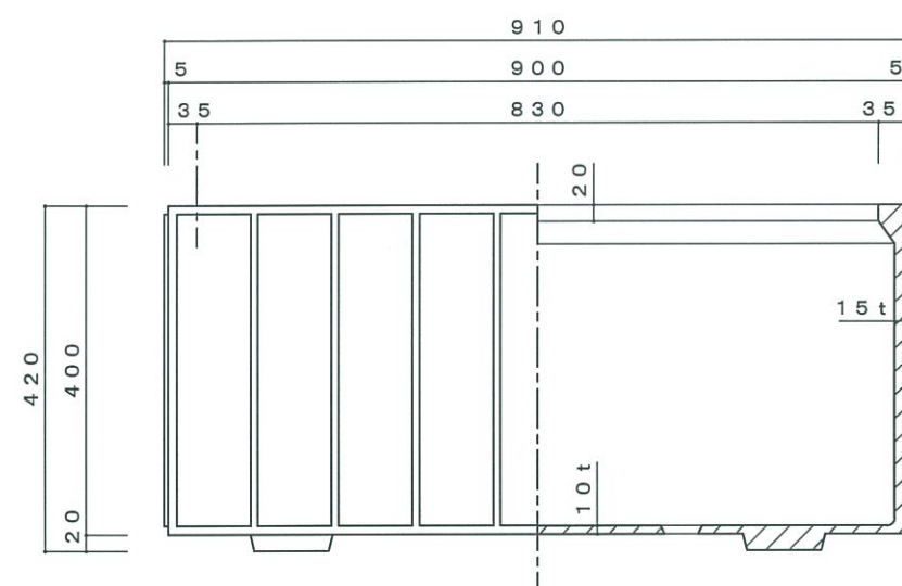
立・断面図
