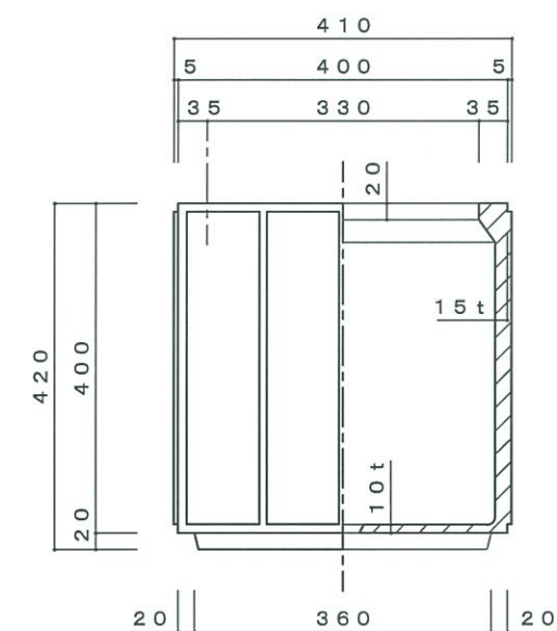
側・断面図
