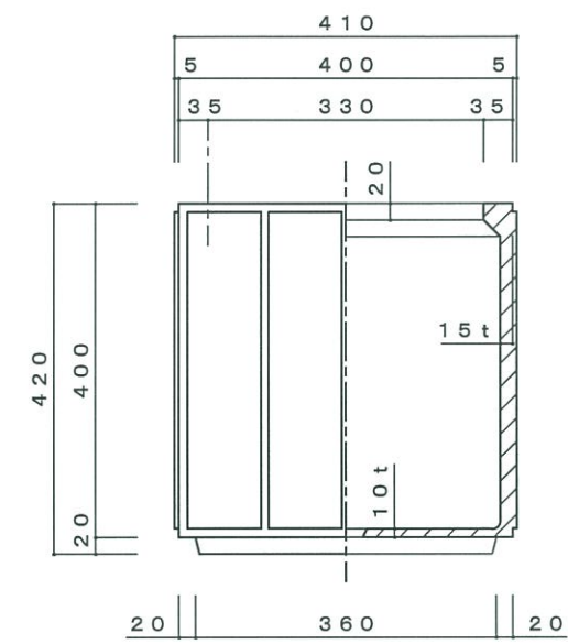
側・断面図
