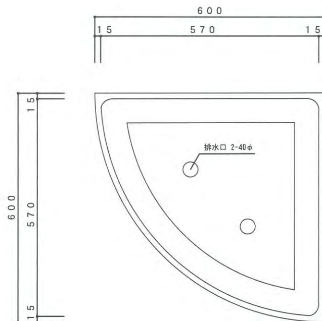
平面図
