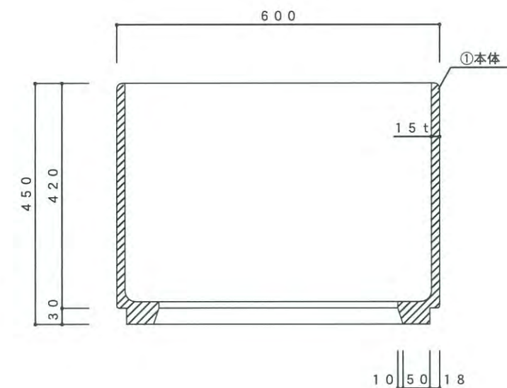
断面図
