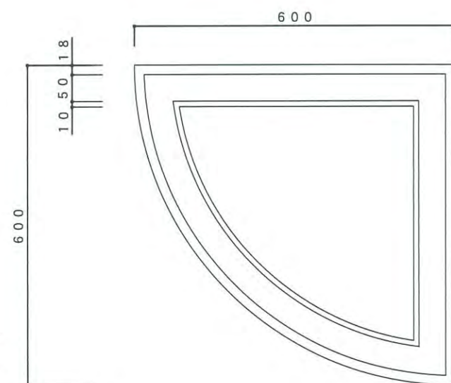
底面図
