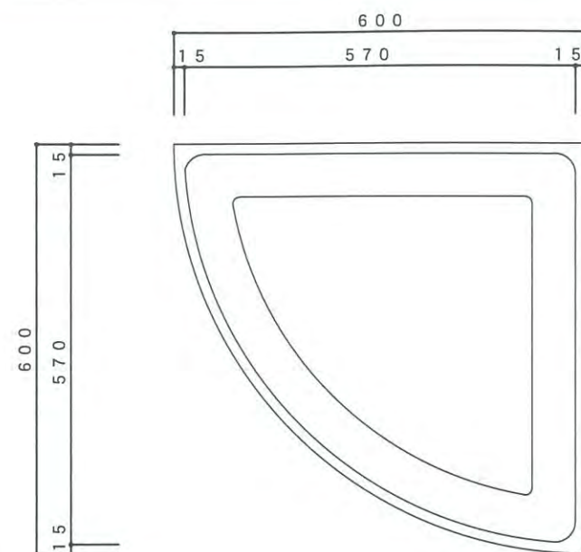
平面図
