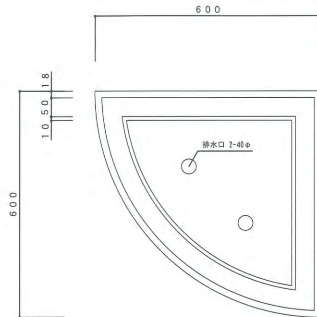
底面図
