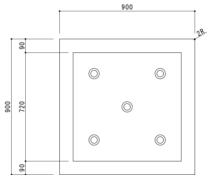
上面図
