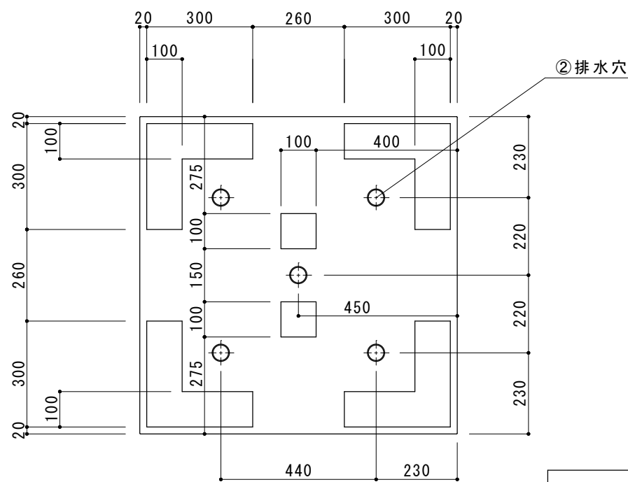
底面図
