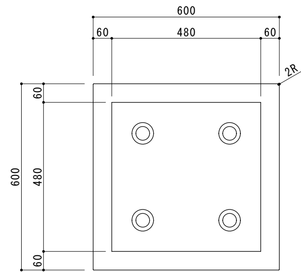
上面図
