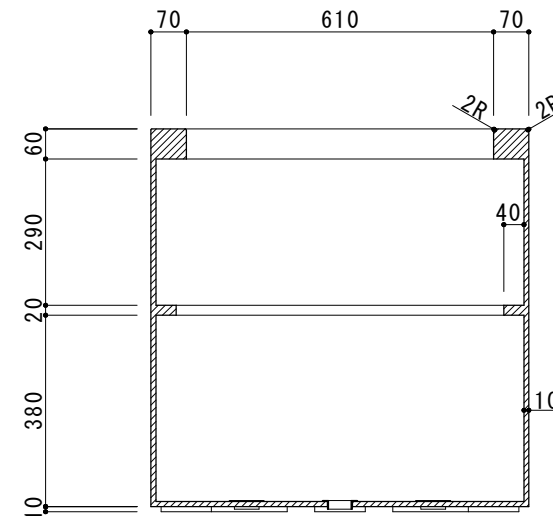
断面図
