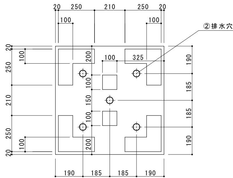
底面図
