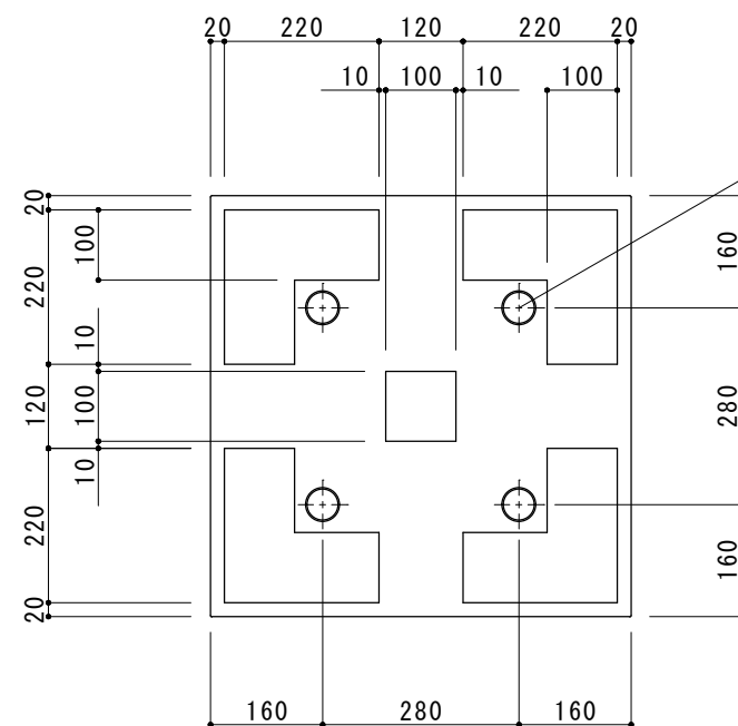
底面図
