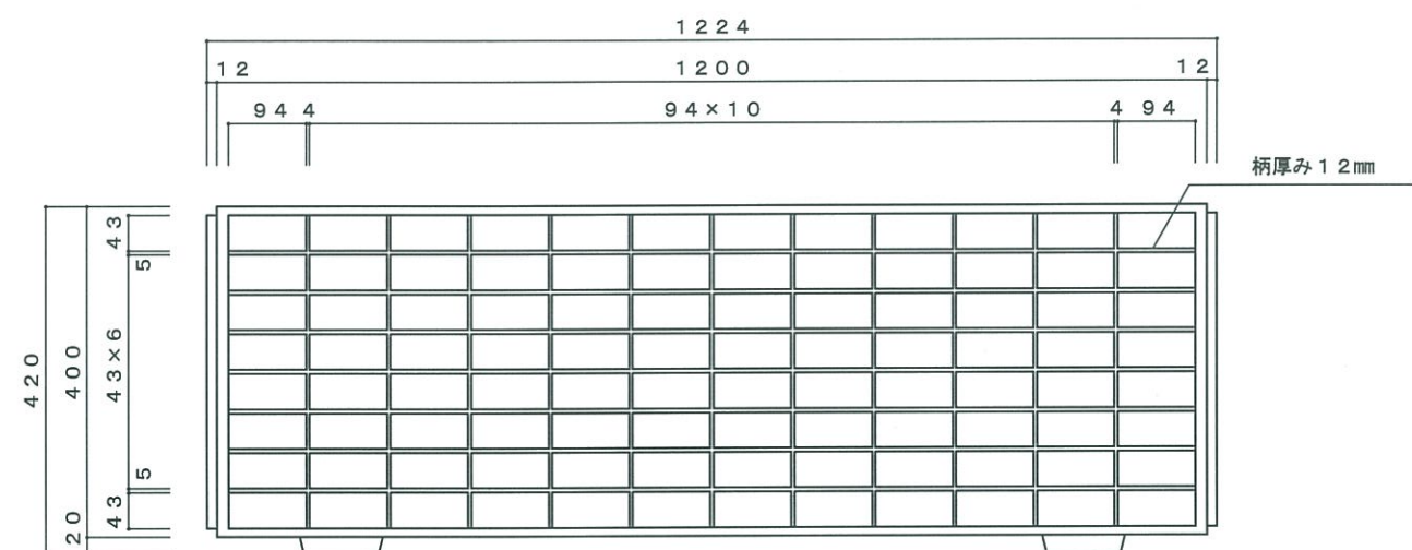
正面図
