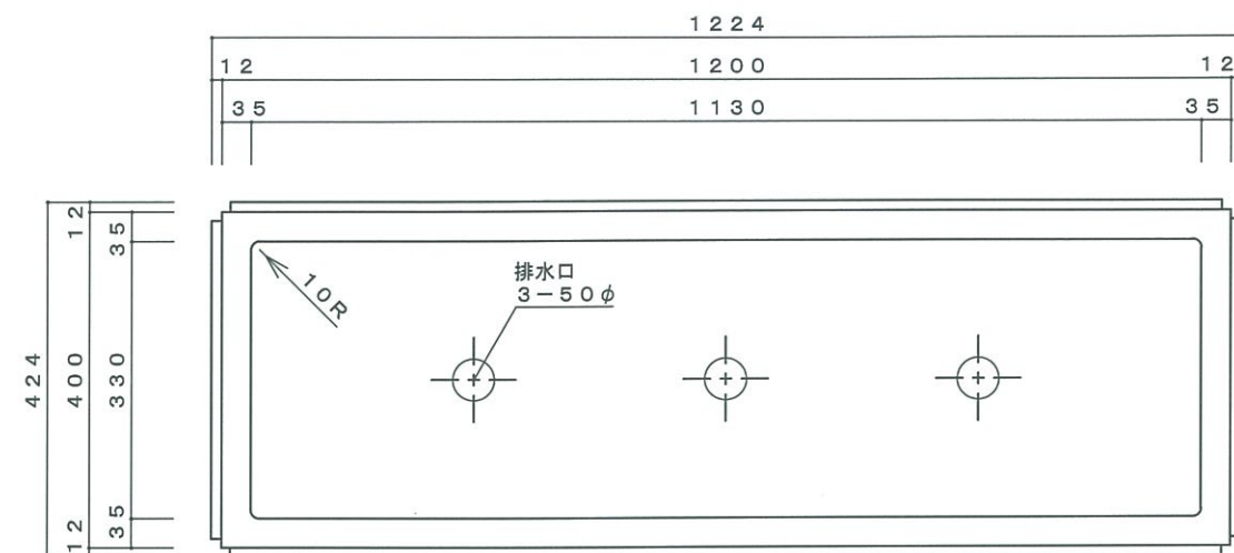
平面図
