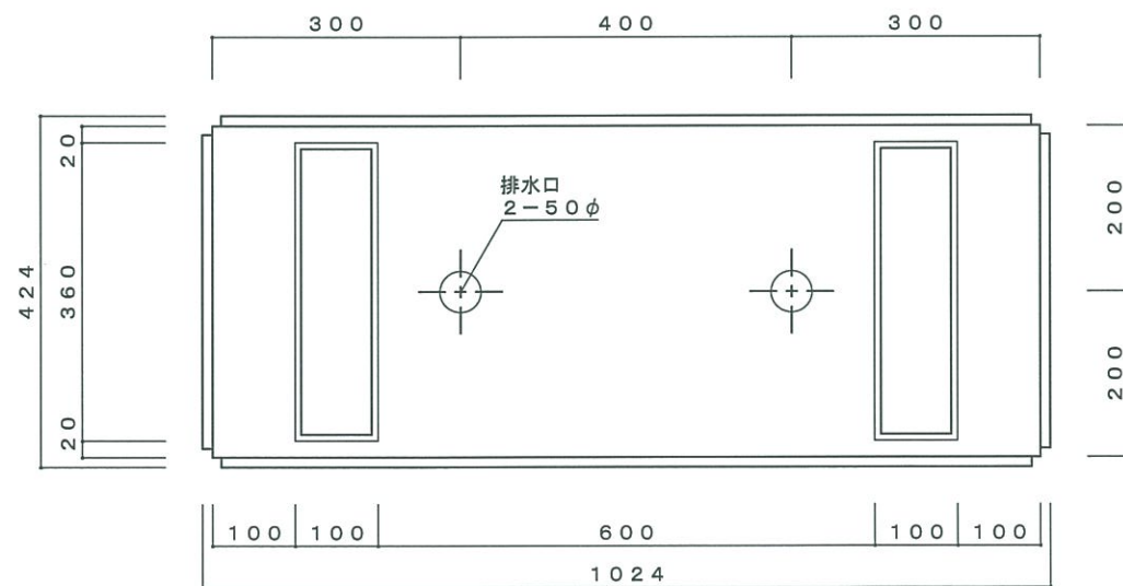
底面図
