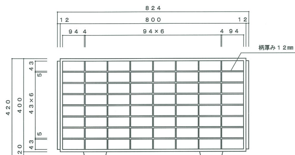
側面図
