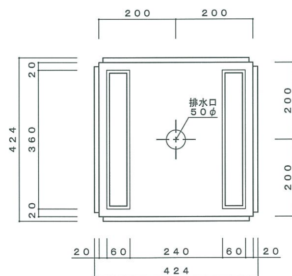
底面図
