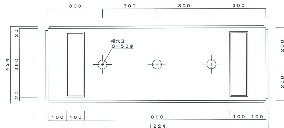
底面図
