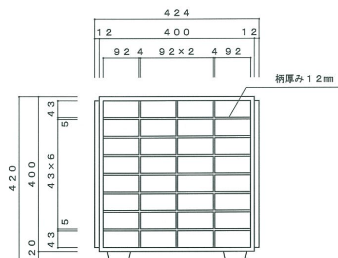
正面図
