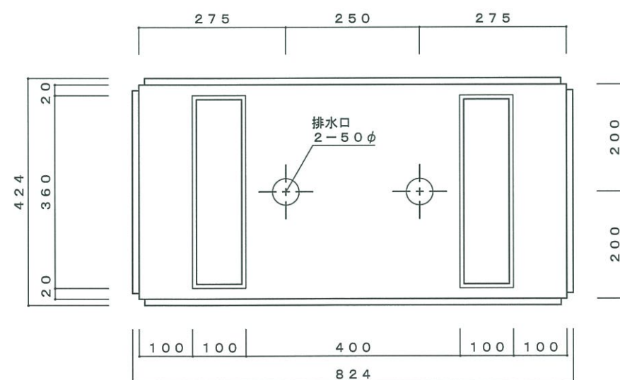
底面図
