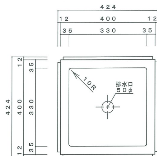
平面図
