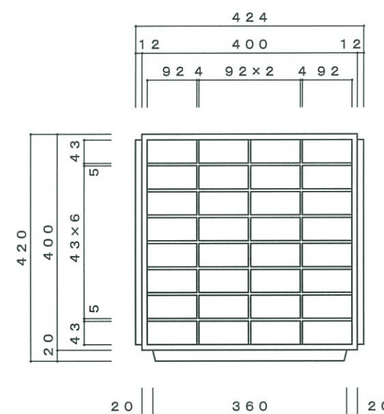
側面図
