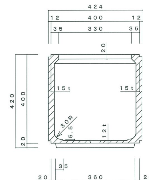
断面図
