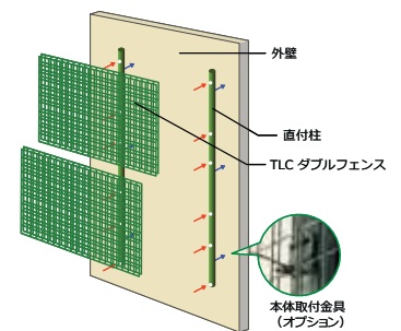
直付柱での取付。
