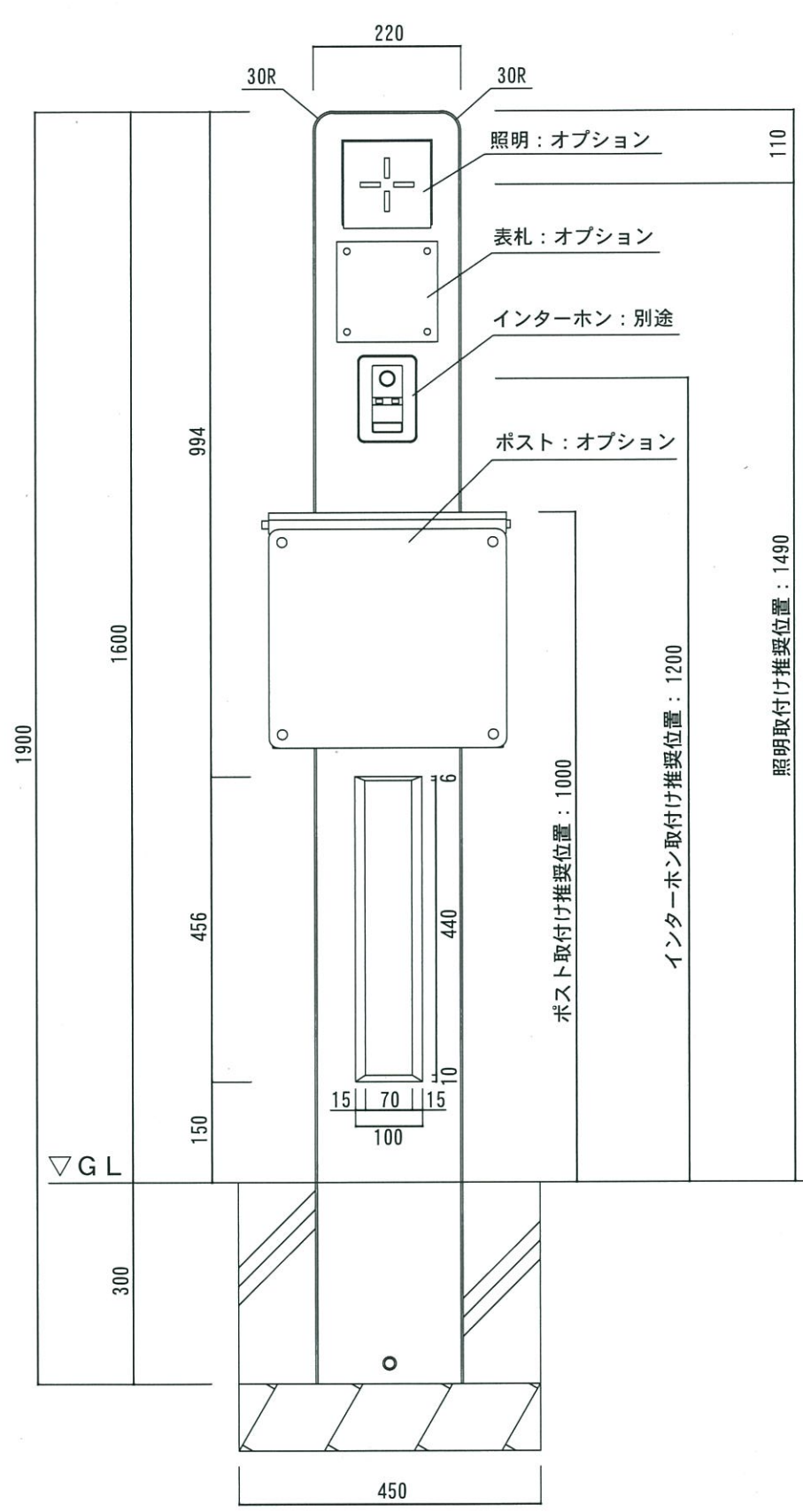
【正面図】
