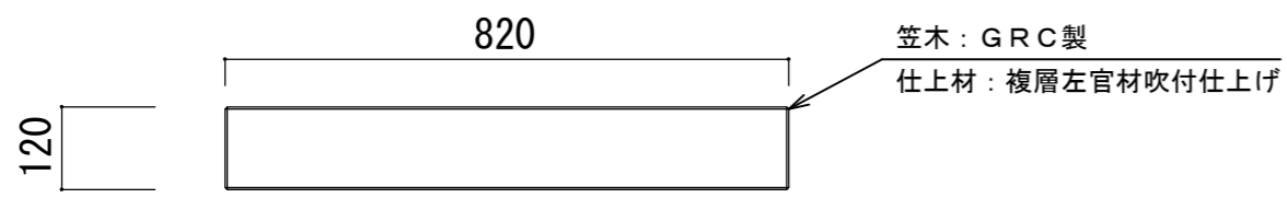
【天面図】
