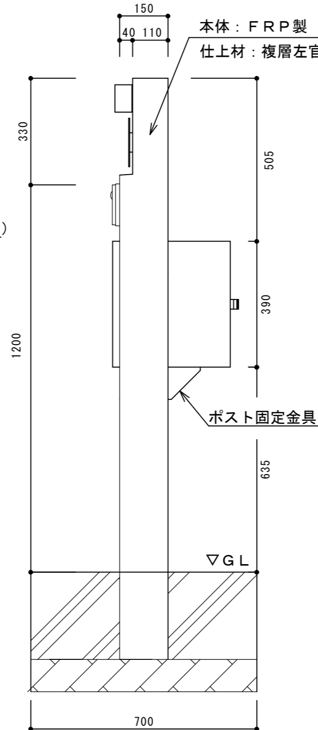
【側面図】
