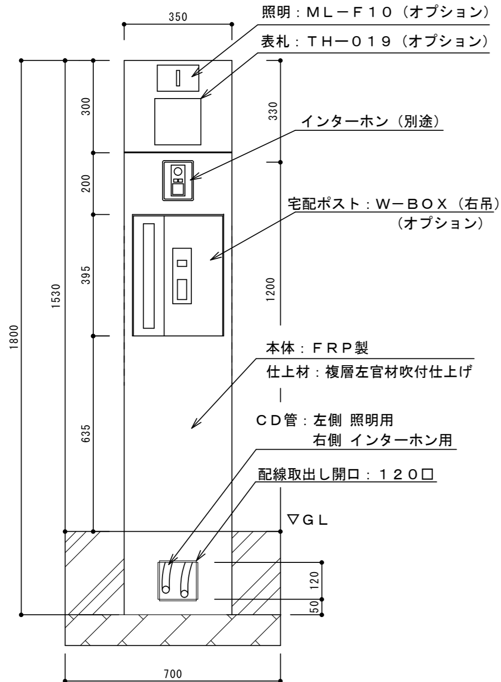
【正面図】
