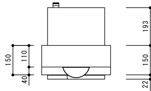
【天面図】
