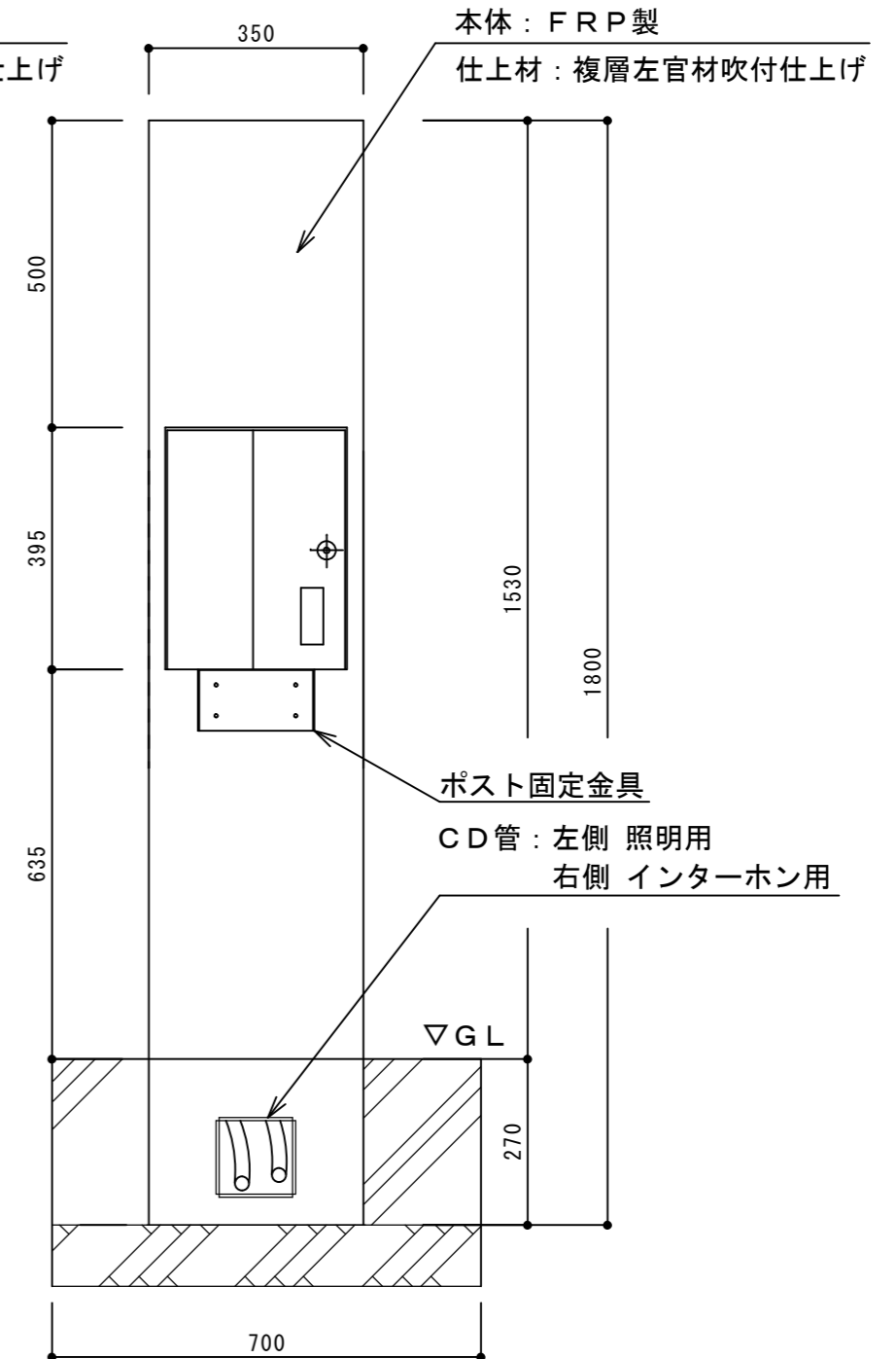
【背面図】
