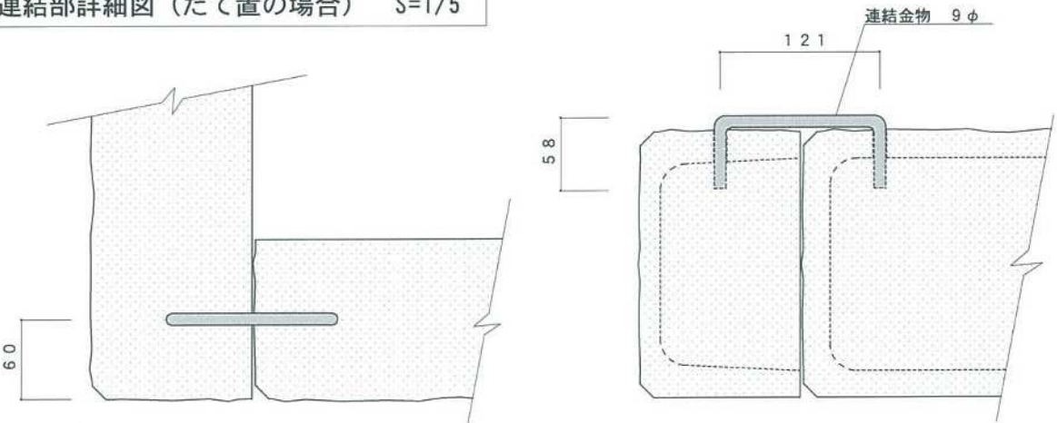
連結部詳細図（たて置の場合） S=1/5
