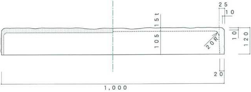
連結部詳細図（たて置の場合） S=1/5
