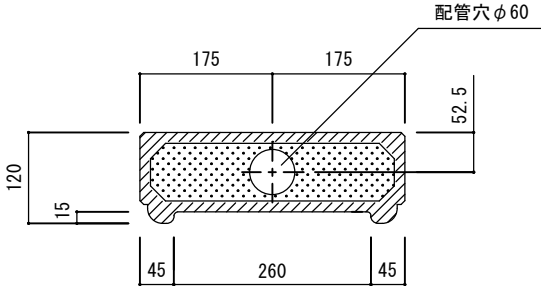
【A-A' 断面図】
