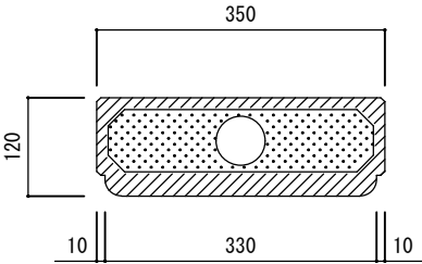
【B-B' 断面図】
