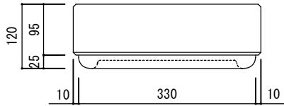
【上面図】
