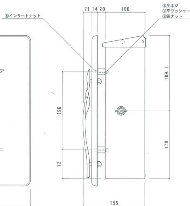
右側面図
