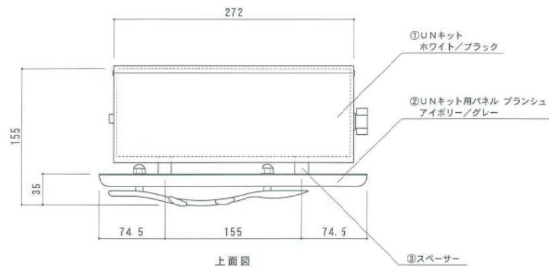
上面図
