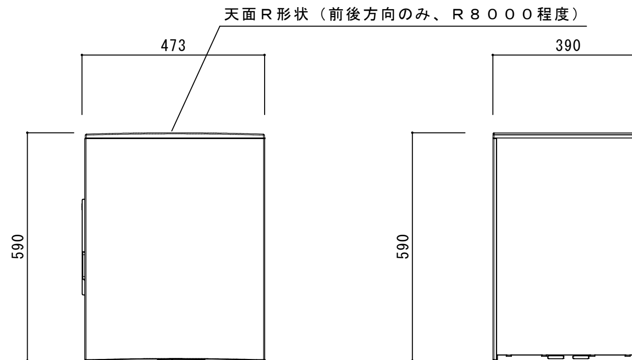
右側面図
