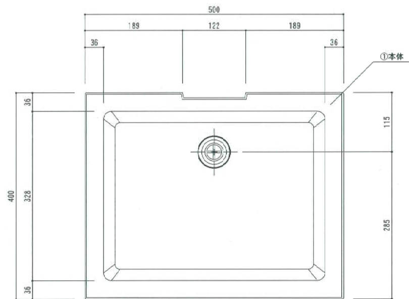
上面図
