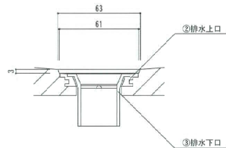
A部詳細図 (S=1/2)
