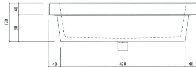
正面図
