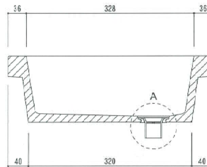
側断面図
