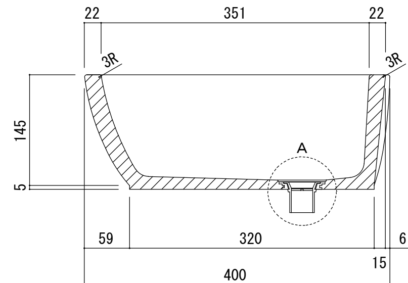
断面図
