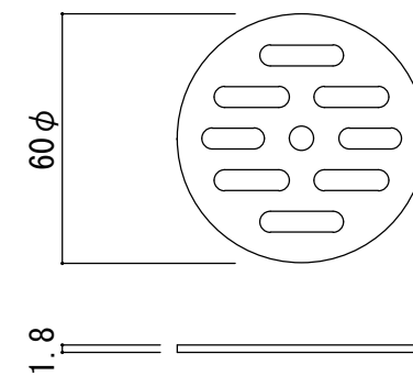
付属品：排水用目皿 (S=1/2)
