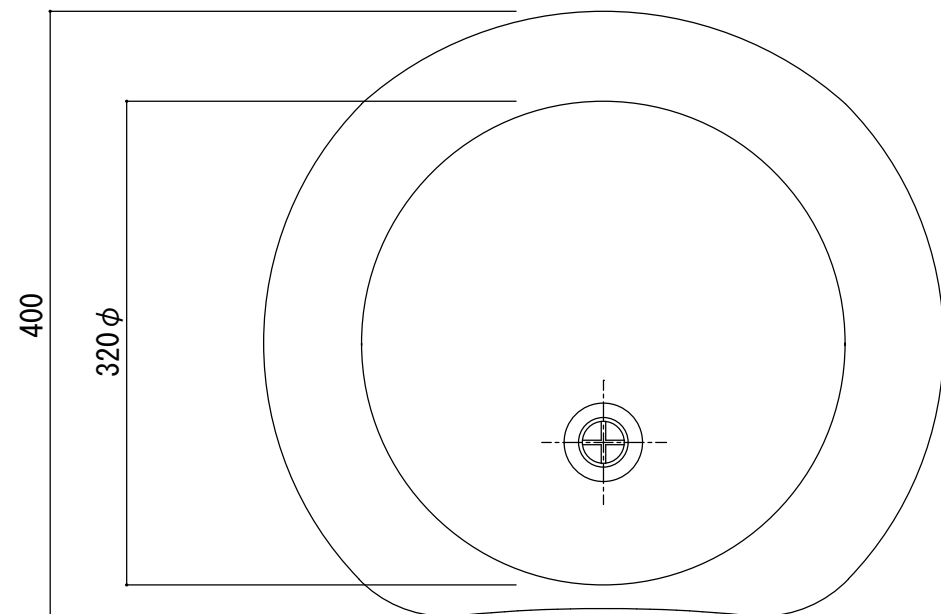
底面図
