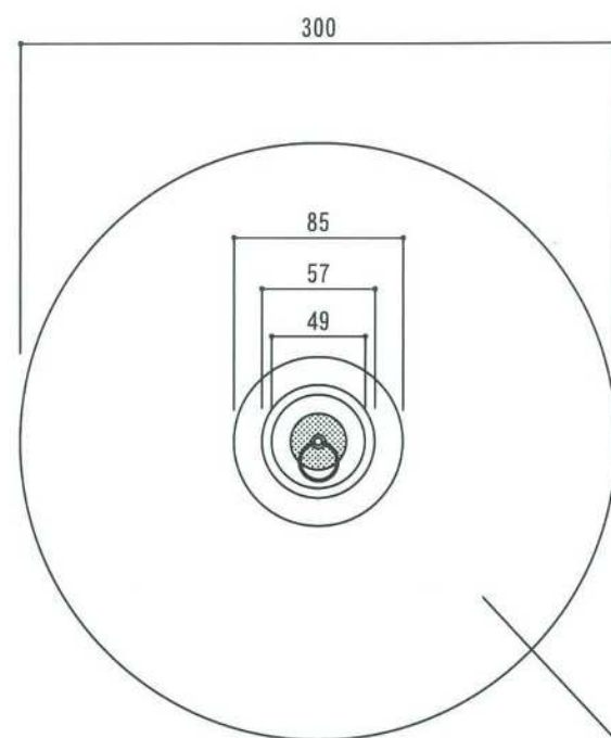
上面図
