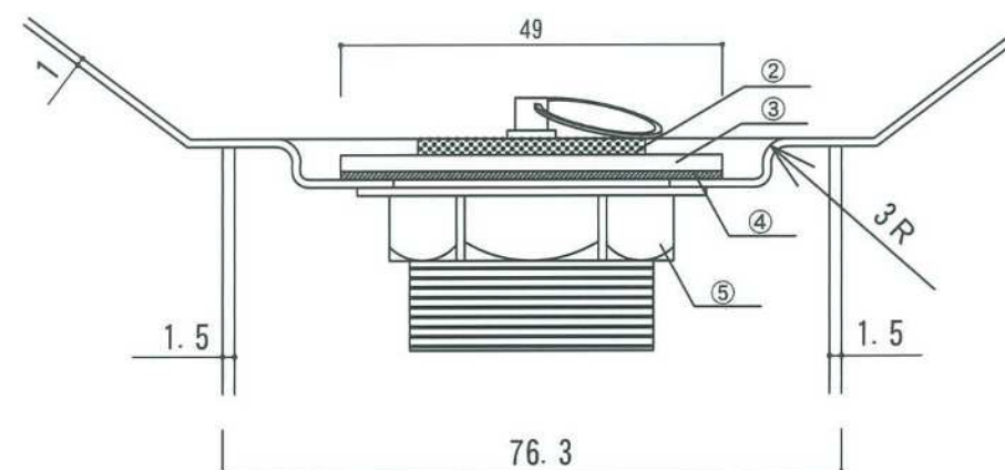
A部拡大 1 / 1
