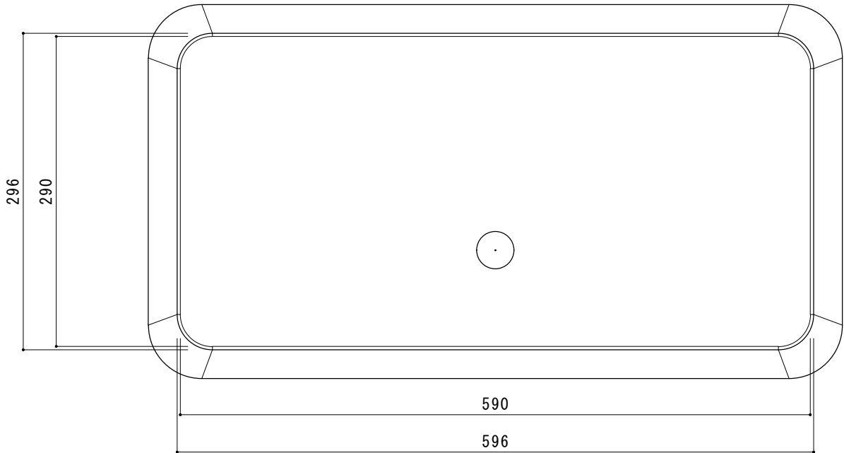
【底面図】
