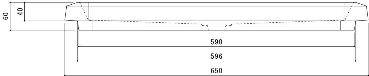
【正面図】
