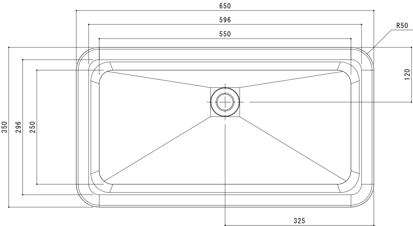
【上面図】
