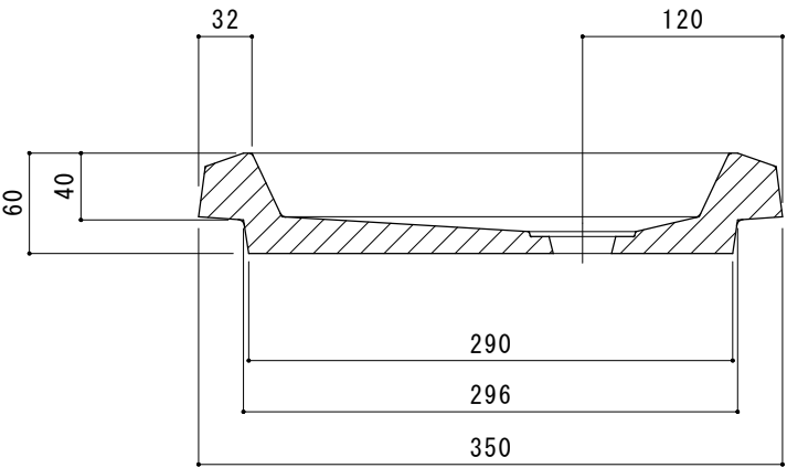
【側面断面図】
