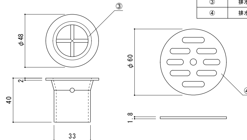
付属品 (S=1/2)
