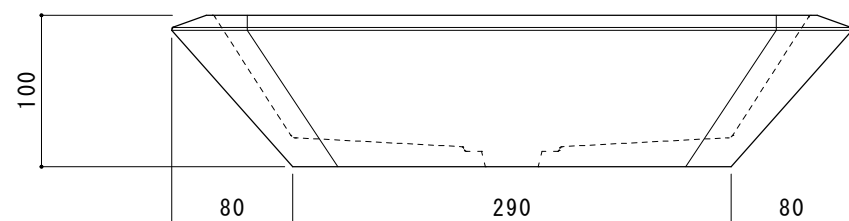
【正面図】
