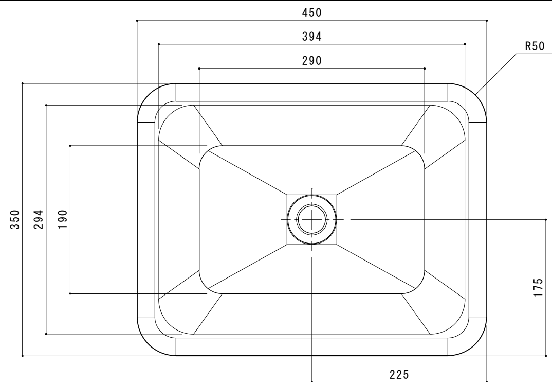
【上面図】
