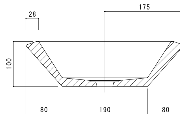
【側面断面図】
