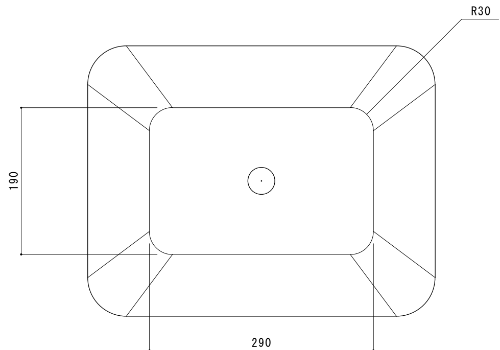
【底面図】
